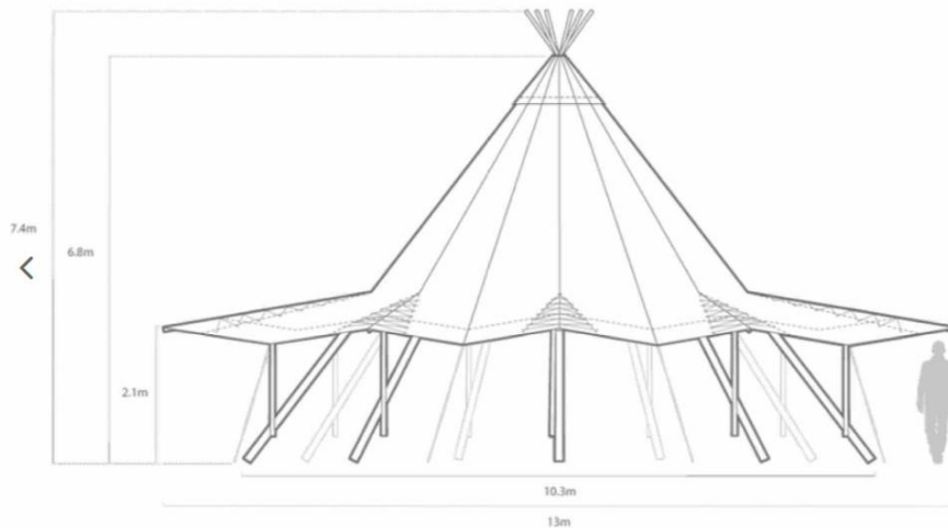
Fig. 2. Billede fra teltudlejningens hjemmeside, luksustelte.dk. Viser skitse af og mål på tipi teltet.
