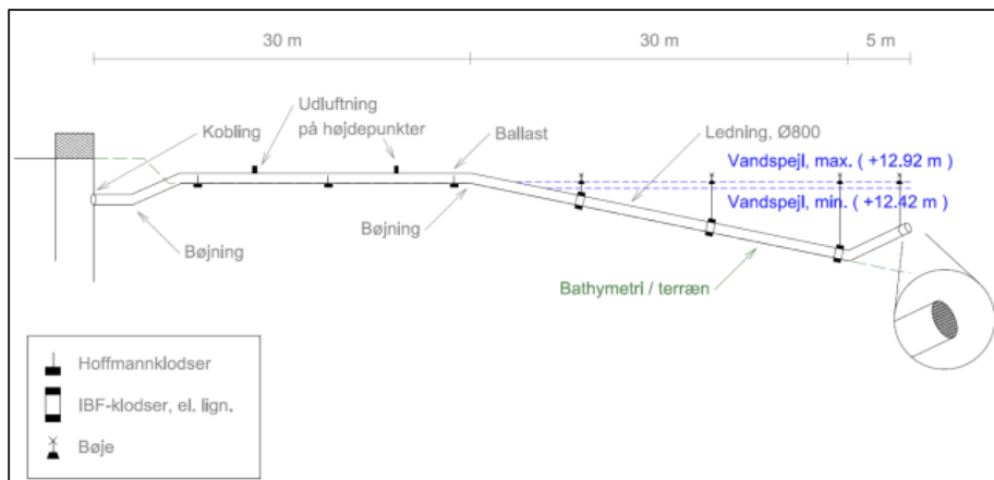
Figur 4. Principskitse for forlængelse af eksisterende udløbsbygværk med et 65 m langt PE-rør ud i Søndersø, så udledningen kommer til at foregå midt i vandsøjlen med en dybde på mellem 2-3 m.
