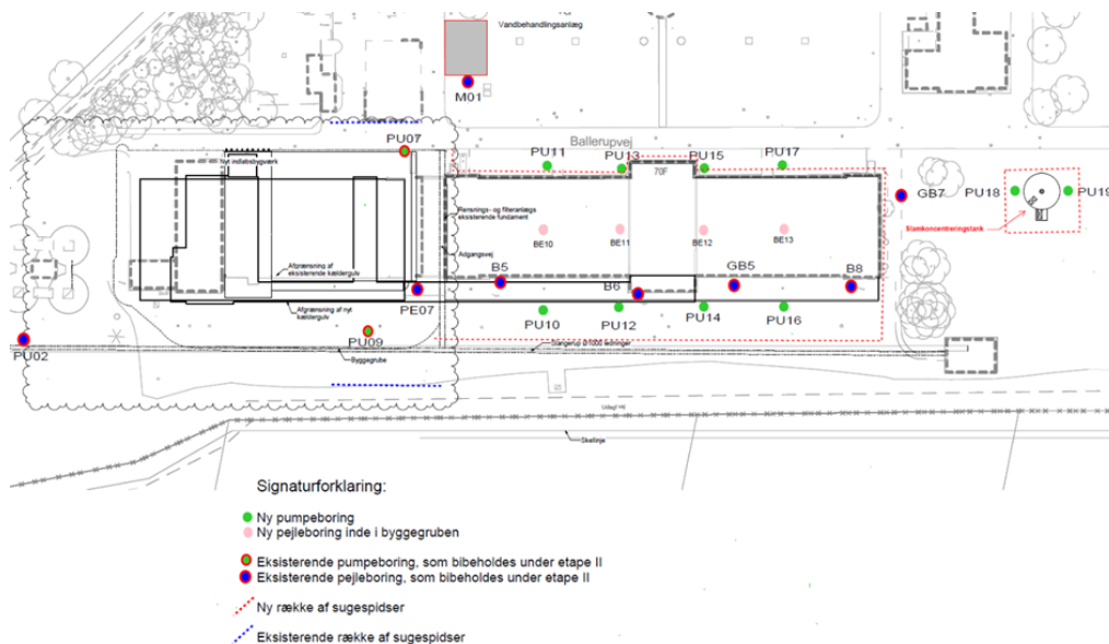
Figur 3. I forbindelse med konstruktion af bygning og kælder i Etape II udføres der grundvandssænkning i byggegruben. På billedet ses forslag til placering af borer og sugespidsler.
