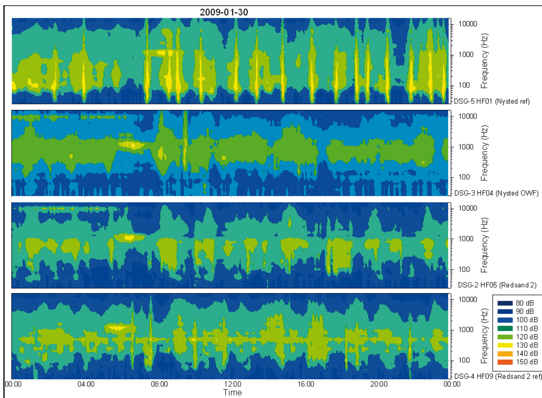
Figur 10 .Tredjedelsoktavspek- tre udregnet løbende hen over et døgn for fire målestationer syd for Rødsand. Støjen er domineret af skibsstøj i om- rådet 100 Hz til ca. 1 kHz. Den øverste station var placeret tæt ved Gedser og her ses tydeligt den regelmæssige signatur af færgen til Rostock. Fra (Teilmann et al, 2009)
