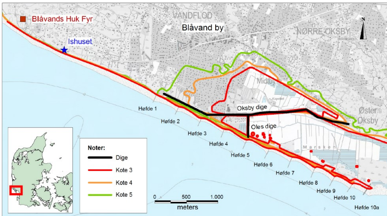
Figur 1. Strækningen, hvor der skal kystbeskyttes ved Blåvand
