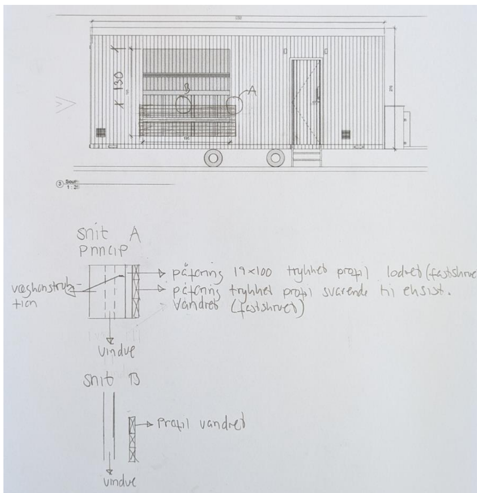
Fig. 6. Tilsendt fra ansøger. På figuren ses en facadetegning af den ansøgte sauna, hvor vinduet er blevet reduceret i størrelse.
