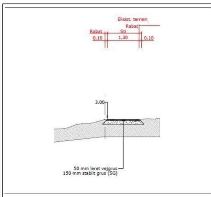
Fig. 9. Skitse af stiens opbygning. Figur fra ansøgningen
