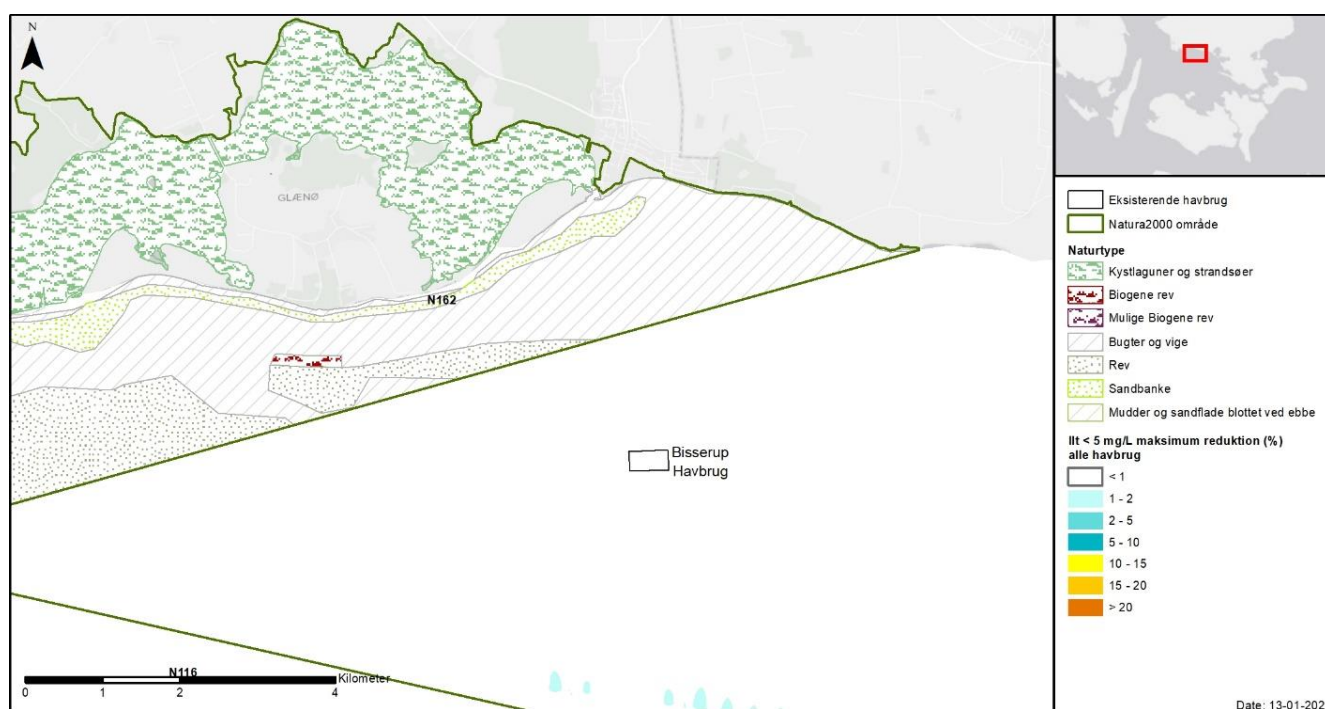
Figur 8-16 Maksimal procentvis ændring i gennemsnitlig ugentlig iltkoncentration ved havbunden ved iltkoncentration < 5 mg L -1 . Bissrup Havbrug kumuleret med omkringliggende havbrug. Ændringer > 10% angiver grænsen for påvirkning foranlediget af ændring i bundvandets koncentration af ilt. Øverst: oversigtskort med Natura 2000-områderne 116, 162, 169 og 173. Nederst: zoom på området omkring Bissrup Havbrug.
