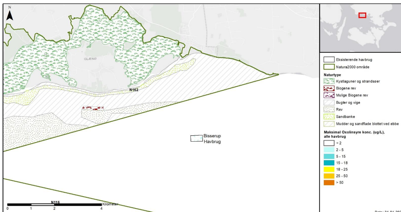
Figur 8-20 Maksimumkoncentrationer af oxolinsyre i overfladen (0-5 m) som følge af samtidig behandling af hele bestanden ved alle 5 havbrug i august. Øverst: oversigtskort med Natura 2000-områderne 116, 162, 169 og 173. Nederst: zoom på området omkring Bissrup Havbrug.
