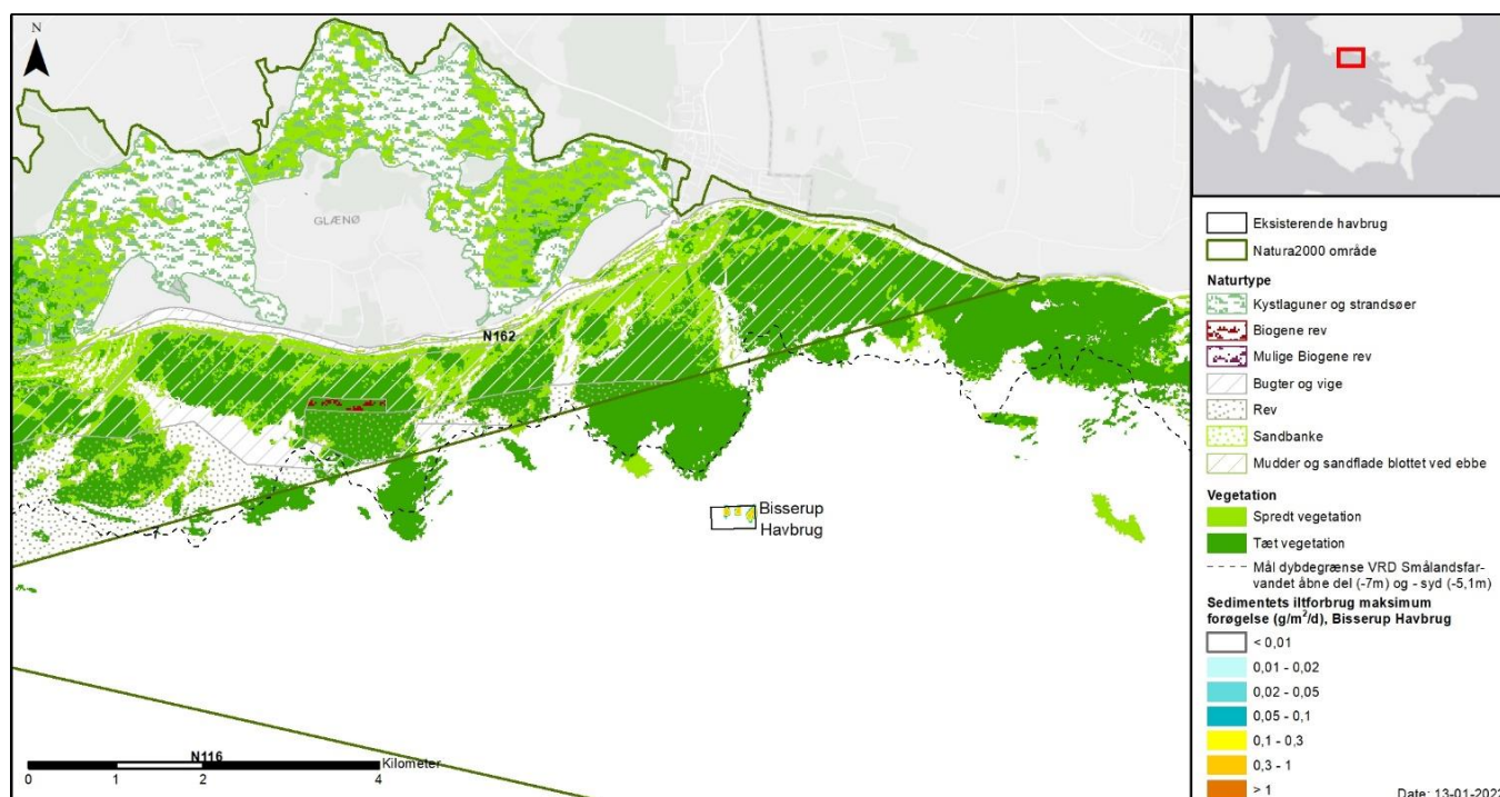
Figur 8-6 Maksimal ændring i gennemsnitligt ugentligt iltforbrug i sedimentet i 5-års perioden for Bisserup Havbrug, i forhold til udbredelsen af bundvegetation (makroalger og ålegræs) opgjort ved satellitdata. Det bemærkes, at satellitdata kun dækker ud til en dybde på 7 m. Maksimal ændring i gennemsnitligt ugentligt iltforbrug > 0,1 \text{ g O}_2 \text{ m}^{-2} \text{ dag}^{-1} angiver grænsen for påvirkning foranlediget af ændringer i sedimentets iltforbrug. Ålegræssets mål-dybdegrænse er angivet som grænseværdier for god-moderat grænsen på hhv. 7 m og 5,1 m i "VRD Smålandsfarvandet åbne del" og "VRD Smålandsfarvandet syd". Øverst: oversigtskort med Natura 2000-områderne 116, 162, 169 og 173. Nederst: zoom på området omkring Bisserup Havbrug.
