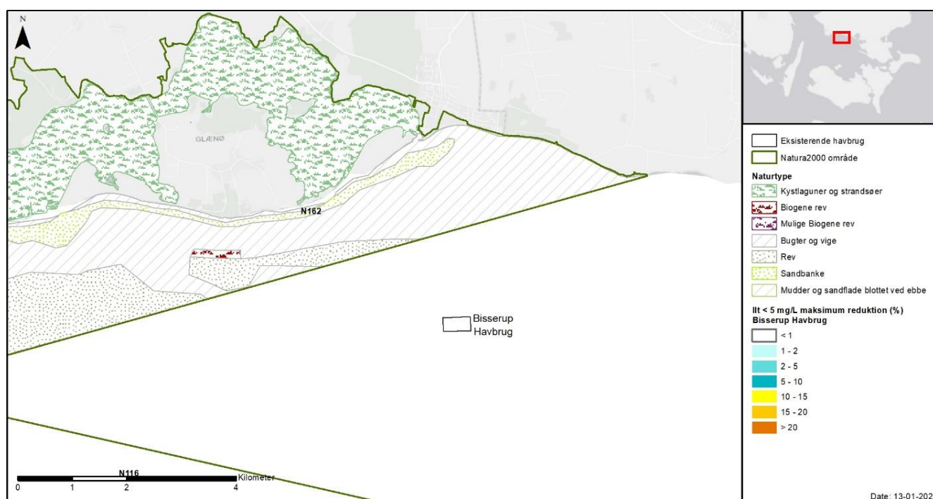
Figur 8-8 Maksimal procentvis ændring i gennemsnitlig ugentlig iltkoncentration ved havbunden (i 5-års perioden) ved iltkoncentration < 5 mg L -1 , for Bissrup Havbrug. Ændringer > 10% angiver grænsen for påvirkning foranlediget af ændring i bundvands koncentration af ilt. Øverst: oversigtskort med Natura 2000-områderne 116, 162, 169 og 173. Nederst: zoom på området omkring Bissrup Havbrug.
