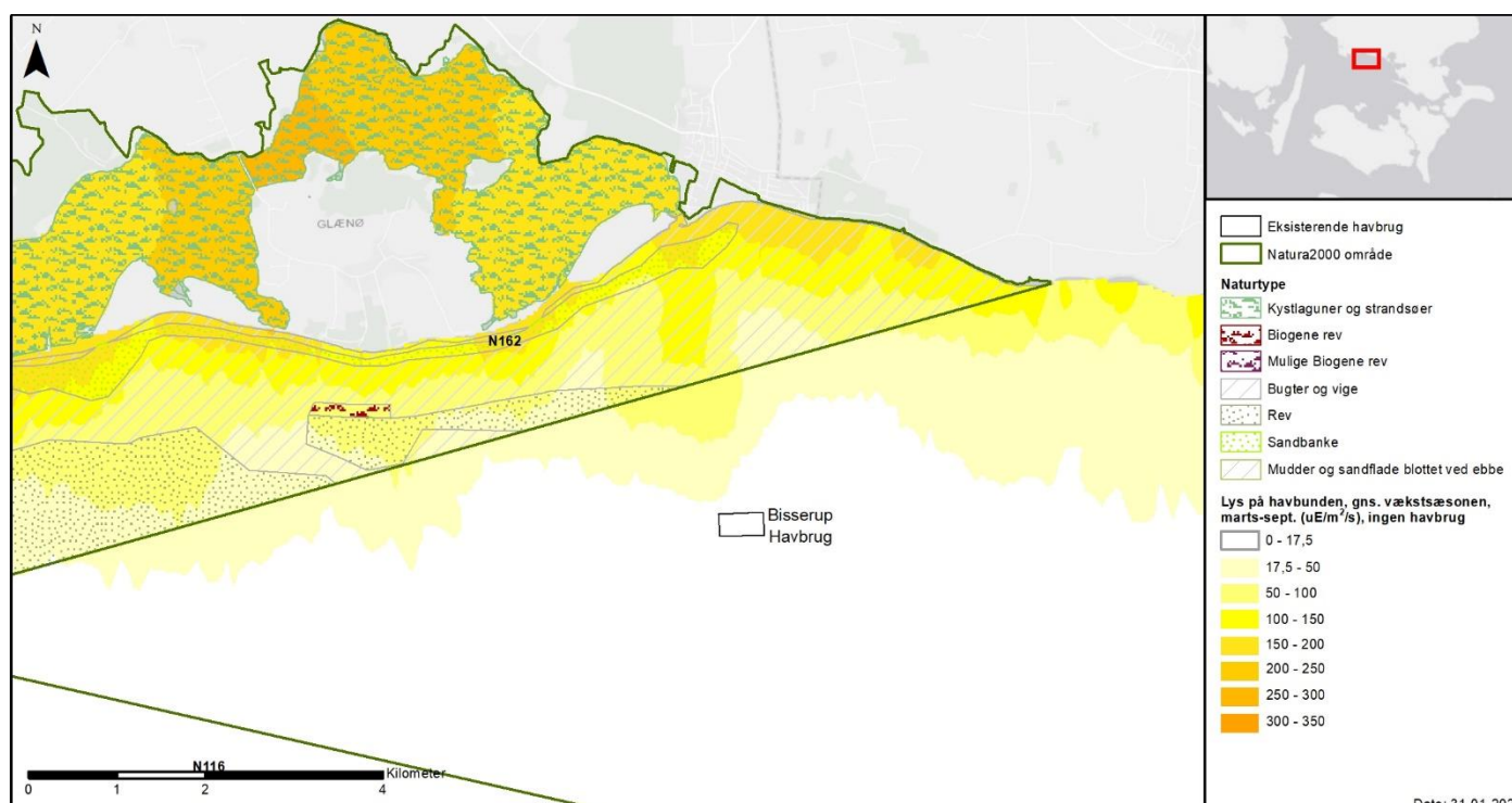
Figur 8-2 Oversigt over gennemsnitligt lys ved havbunden ( \mu E m^{-2} s^{-1} ) i bundplanternes vækstsæson fra marts - september i perioden 2014-2018. Øverst: oversigtskort med Natura 2000-områderne 116, 162, 169 og 173. Nederst: zoom på området omkring Bissrup Havbrug.
