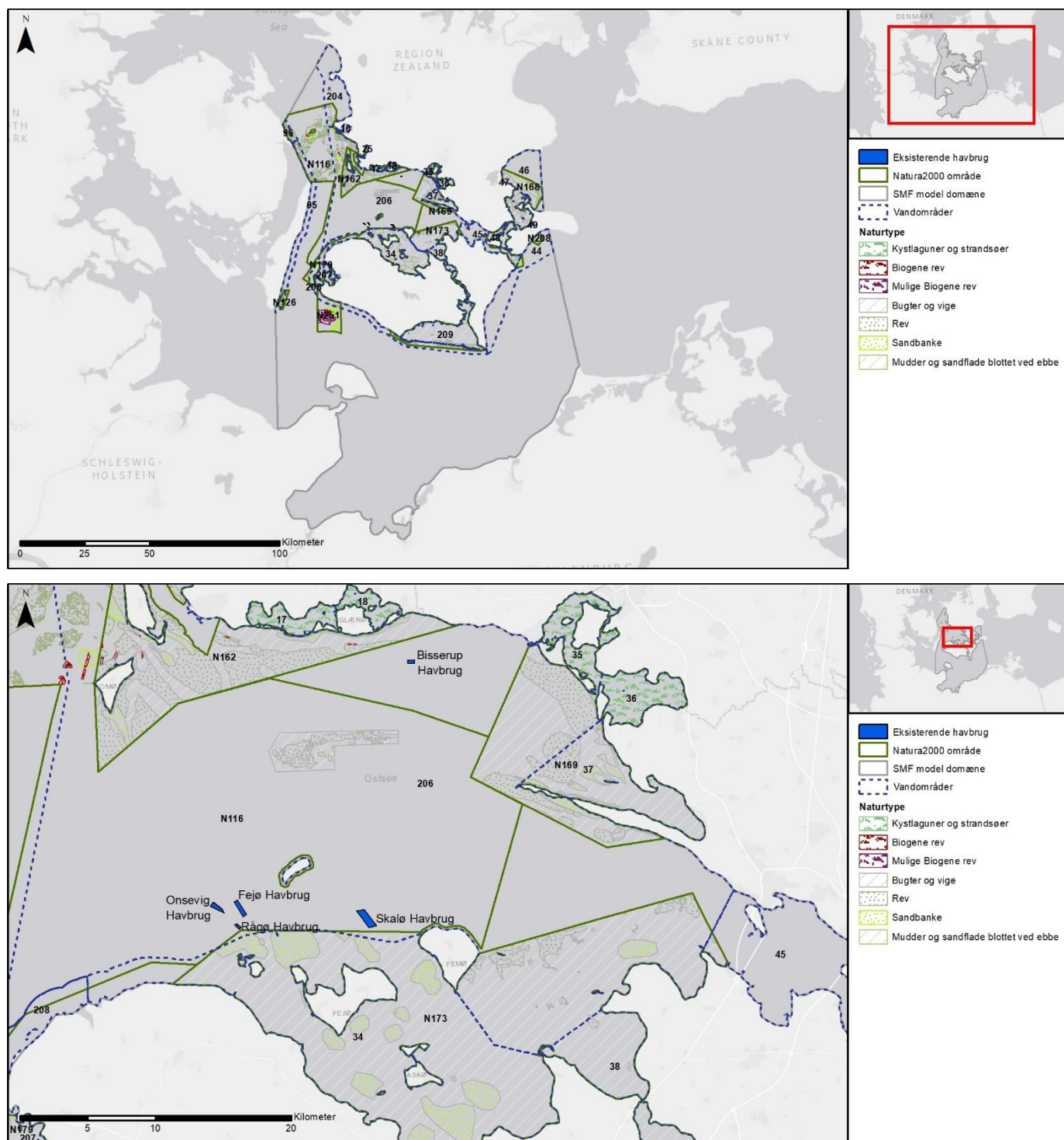
Figur 3-1 Placering af Bissrup Havbrug i forhold til Natura 2000-områder og vandplansområder (angivet med område ID).
