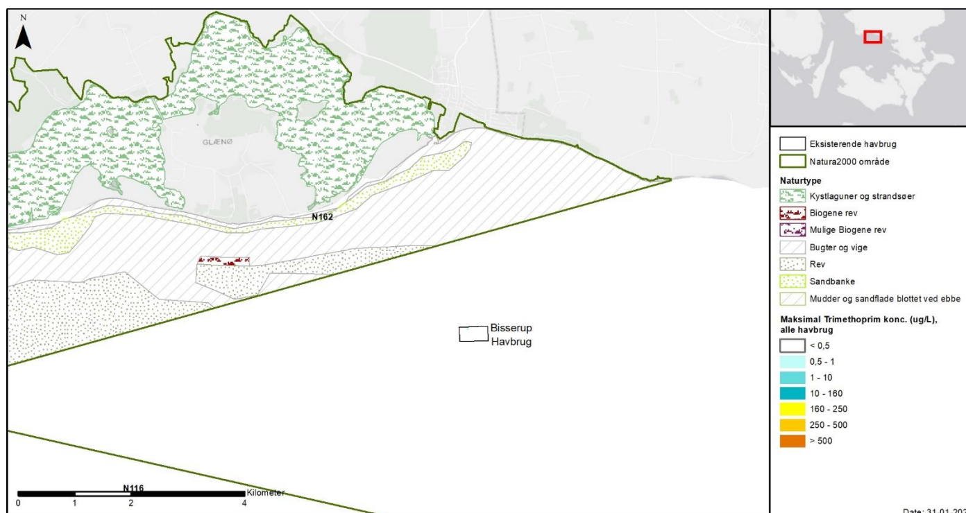
Figur 8-23 Maksimumkoncentrationer af trimethoprim i overfladen (0-5 m) som følge af samtidig behandling af hele bestanden ved alle 5 havbrug i august. Øverst: oversigtskort med Natura 2000-områderne 116, 162, 169 og 173. Nederst: zoom på området omkring Bissrup Havbrug.
