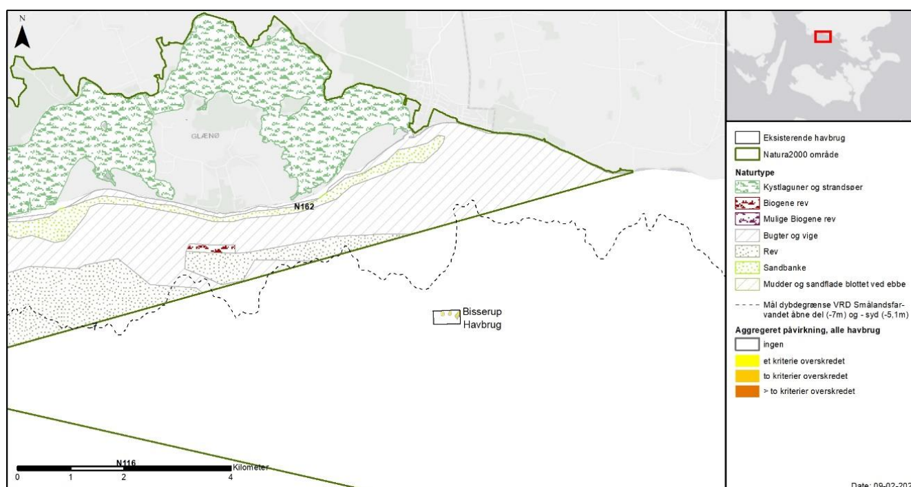
Figur 8-18 Aggregeret påvirkning identificeret ved de fire vurderingskriterier foranlediget af produktionen ved Bissrup, Onsevig, Rågø, Fejø og Skalø Havbrug kumulativt. Ålegræssets mål-dybdegrænse er angivet som grænseværdier for god-moderat grænsen på hhv. 7 m og 5,1 m i "VRD Smålandsfarvandet åbne del" og "VRD Smålandsfarvandet syd". Øverst: oversigtskort med Natura 2000-områderne 116, 162, 169 og 173. Nederst: zoom på området omkring Bissrup Havbrug.
