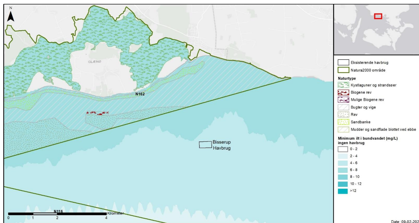
Figur 8-3 Oversigt over minimum ilt i bundvandet ( \text{mg L}^{-1} ) i perioden 2014-2018. Øverst: oversigtskort med Natura 2000-områderne 116, 162, 169 og 173. Nederst: zoom på området omkring Bissrup Havbrug.
