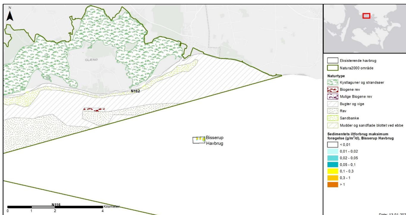
Figur 8-5 Maksimal ændring i gennemsnitligt ugentligt iltforbrug i sedimentet i 5-års perioden i forhold til naturtyper for Bissrup Havbrug. Maksimal øgning i gennemsnitligt ugentligt iltforbrug > 0,1 \text{ g O}_2 \text{ m}^{-2} \text{ dag}^{-1} angiver grænsen for påvirkning foranlediget af ændringer i sedimentets iltforbrug. Øverst: oversigtskort med Natura 2000-områderne 116, 162, 169 og 173. Nederst: zoom på området omkring Bissrup Havbrug.
