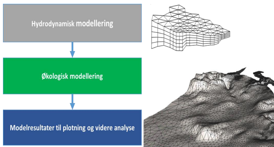
Figur 7-2 Opbygning af modelkomplekset. Tv. modelleringprocessen. Th. illustration af modelkompleksets opdeling i FM (flexible mesh) celler øverst eksempel på opdeling i vandfasen nederst eksempel på, hvordan nettet ser ud på havbunden og havbund-topologien i en model (ikke fra den aktuelle model). I korte tidsskridt (sekunder) beregnes resultatet af de hydrodynamiske og økologiske processer og interaktioner i og mellem cellerne.
