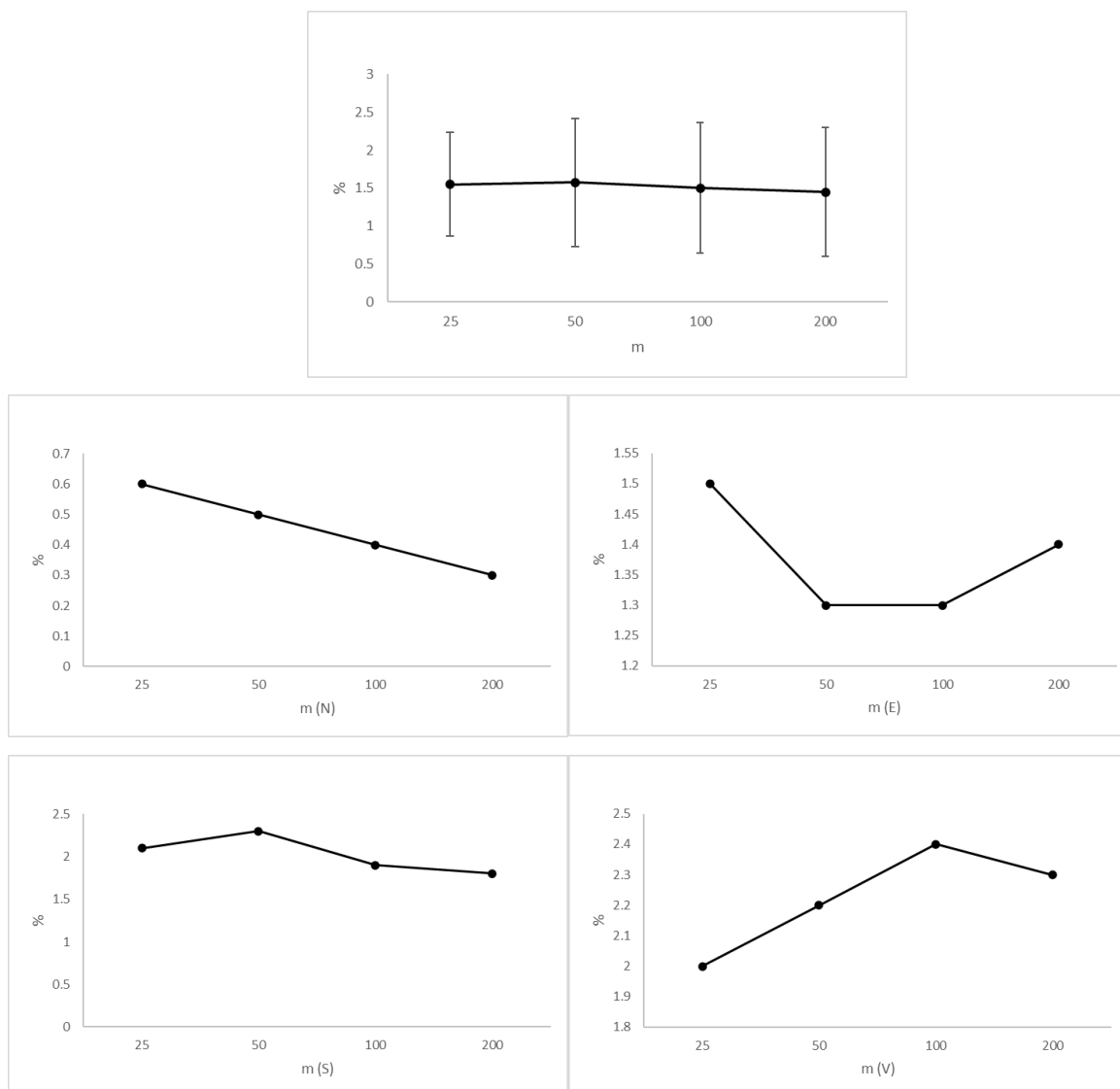
Figur 8-38 Glødetab i sedimentet ved og omkring Bissrup Havbrug. Gennemsnit og standardafvigelse af glødetabet (øverst) og observeret gødetab N (25-200 m), Ø (25-200 m), S (25-200 m) og V (25-200 m) for havbruget.
