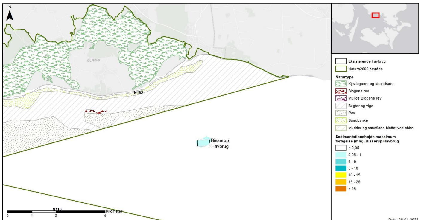
Figur 8-4 Maksimal tilføjede sedimentationshøjde (mm) ved og omkring Bissrup Havbrug i 5- års perioden. Sedimentationshøjde på > 10 mm angiver grænsen for mekanisk påvirkning foranlediget af sedimentation af organisk materiale. Øverst: oversigtskort med Natura 2000-områderne 116, 162, 169 og 173. Nederst: zoom på området omkring Bissrup Havbrug.
