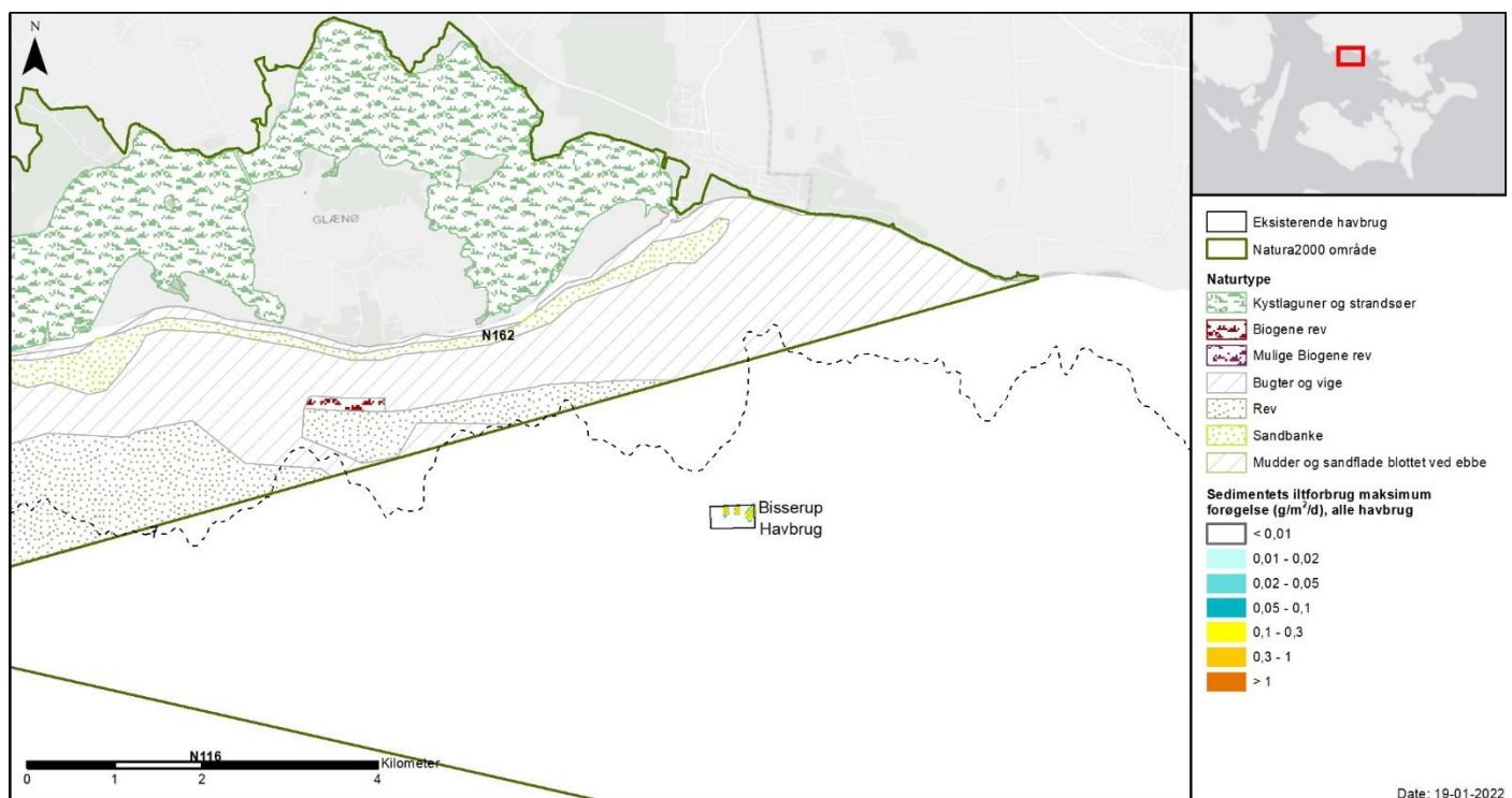
Figur 8-12 Maksimal ændring i gennemsnitligt, ugentligt iltforbrug i sedimentet, Bissrup Havbrug kumuleret med omkringliggende havbrug. Ændring i gennemsnitligt, ugentligt iltforbrug > 0,1 \text{ g O}_2 \text{ m}^{-2} \text{ dag}^{-1} angiver grænsen for påvirkning foranlediget af ændringer i sedimentets iltforbrug. Øverst: oversigtskort med Natura 2000-områderne 116, 162, 169 og 173. Nederst: zoom på området omkring Bissrup Havbrug.
