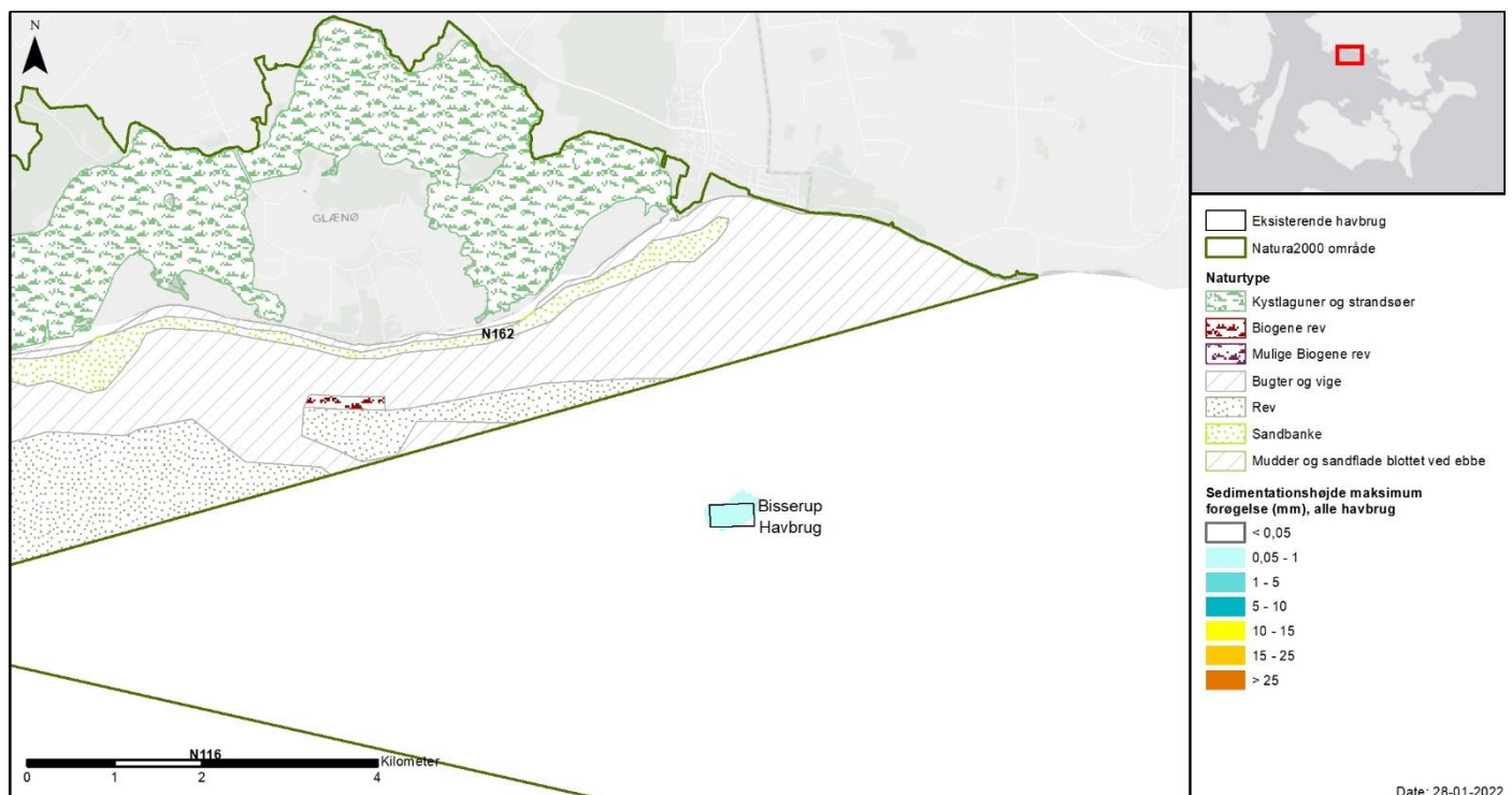
Figur 8-11 Maksimal tilføjede sedimentationshøjde, Bissrup Havbrug kumuleret med omkringliggende havbrug. Sedimentationshøjde på > 10 mm angiver grænsen for mekanisk påvirkning foranlediget af sedimentation af organisk materiale. Øverst: over-sigtskort med Natura 2000-områderne 116, 162, 169 og 173. Nederst: zoom på området omkring Bissrup Havbrug.
