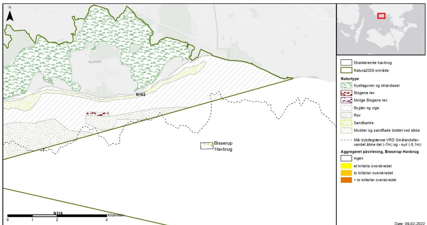
Figur 8-10 Aggregeret påvirkning identificeret ved de fire vurderingskriterier, opgjort for Bissrup Havbrug. Ålegræssets mål-dybdegrænse er angivet som grænseværdier for god-moderat grænsen på hhv. 7 m og 5,1 m i "VRD Smålandsfarvandet åbne del" og "VRD Smålandsfarvandet syd". Øverst: oversigtskort med Natura 2000-områderne 116, 162, 169 og 173. Nederst: zoom på området omkring Bissrup Havbrug.
