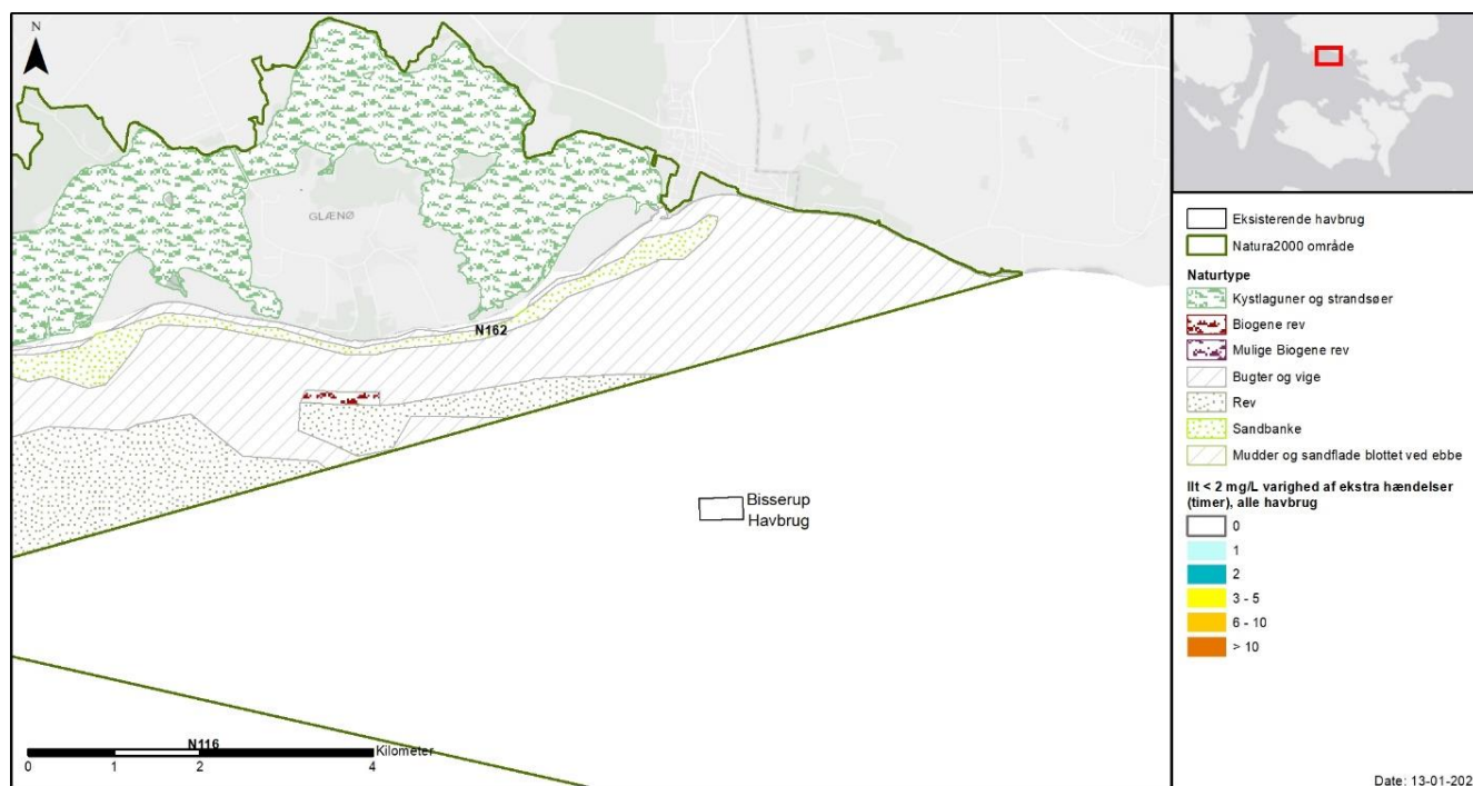
Figur 8-17 Varighed af ekstra hændelser med lave ( < 2 \text{ mg L}^{-1} ) iltkoncentrationer i bundvandet. Bissrup Havbrug kumuleret med omkringliggende havbrug. Ændringer med varighed > 2 timer angiver grænsen for påvirkning foranlediget af ændring i bundvandets koncentration af ilt. Øverst: oversigtskort med Natura 2000-områderne 116, 162, 169 og 173. Nederst: zoom på området omkring Bissrup Havbrug.
