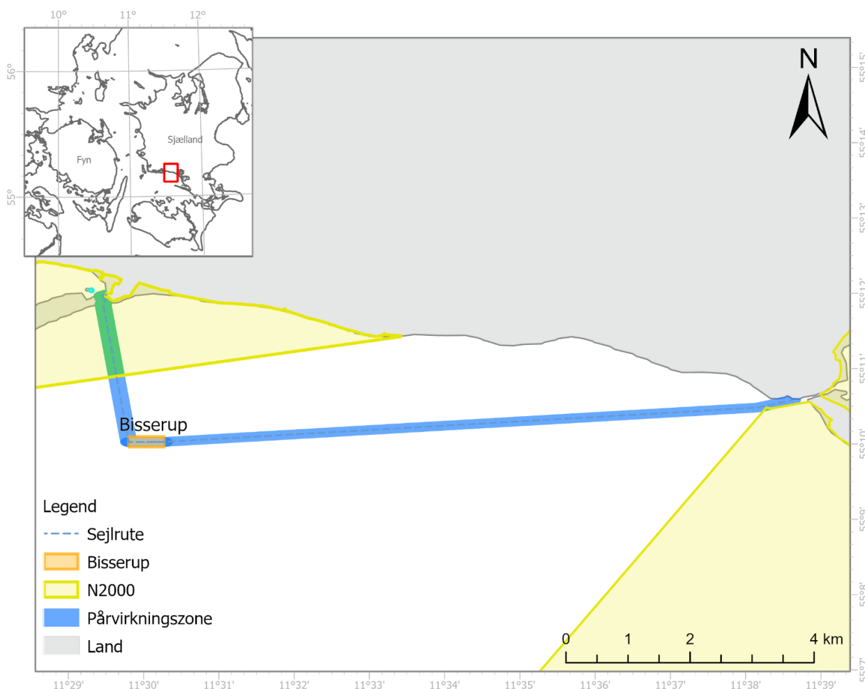
Figur 8-37 Påvirkningszoner for Bissrup Havbrug. Stiplet linje angiver sejlrouterne fra Bissrup Havn og Karrebæksminde Havn til Bissrup Havbrug. Den blå polygon angiver den effektive påvirkningszone (2*120 m), som er grøn ved overlap med N162 og N169 (nord og øst for Bissrup Havbrug).
