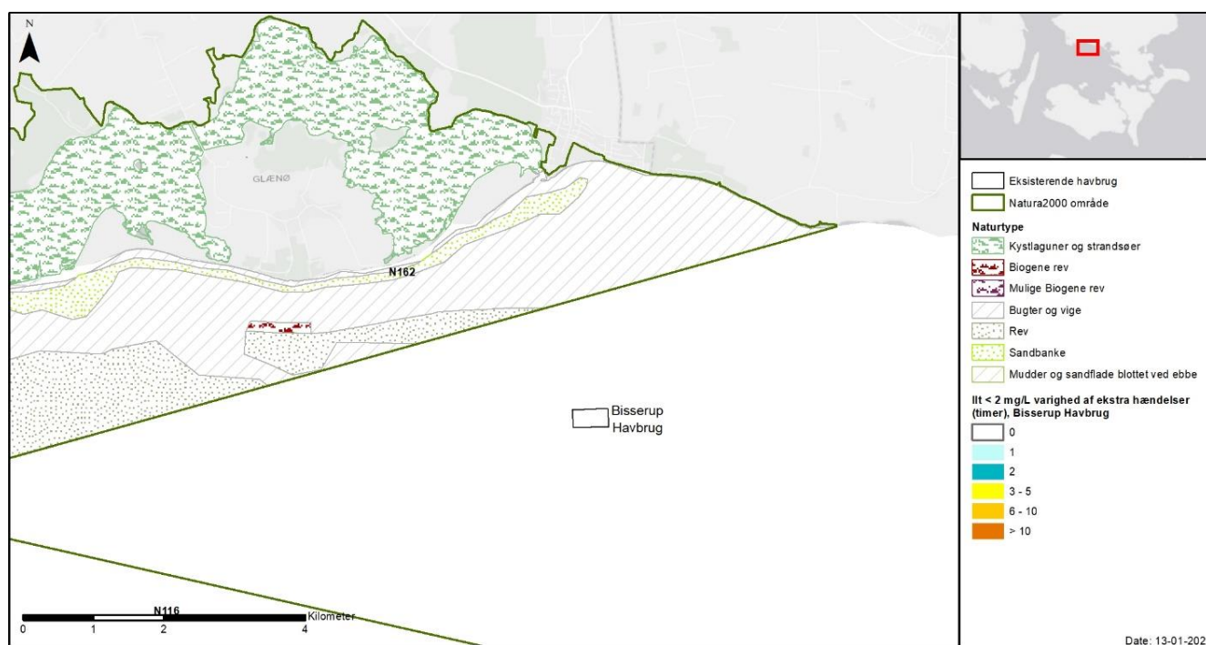
Figur 8-9 Varighed af ekstra hændelser med lave ( < 2 \text{ mg L}^{-1} ) iltkoncentrationer i bundvandet (i 5-års perioden) for Bissrup Havbrug. Ændringer med varighed > 2 timer angiver grænsen for påvirkning foranlediget af ændring i bundvandets koncentration af ilt. Øverst: oversigtskort med Natura 2000-områderne 116, 162, 169 og 173. Nederst: zoom på området omkring Bissrup Havbrug.
