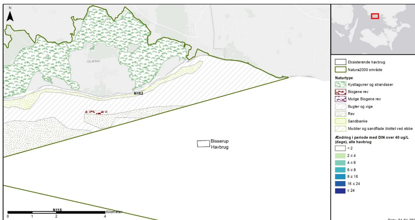
Figur 8-19 Varighed af ekstra hændelser med DIN > 40 µg L -1 i bundvandet. Bissrup Havbrug kumuleret med omkringliggende havbrug. Øverst: oversigtskort med Natura 2000-områderne 116, 162, 169 og 173. Nederst: zoom på området omkring Bissrup Havbrug.
