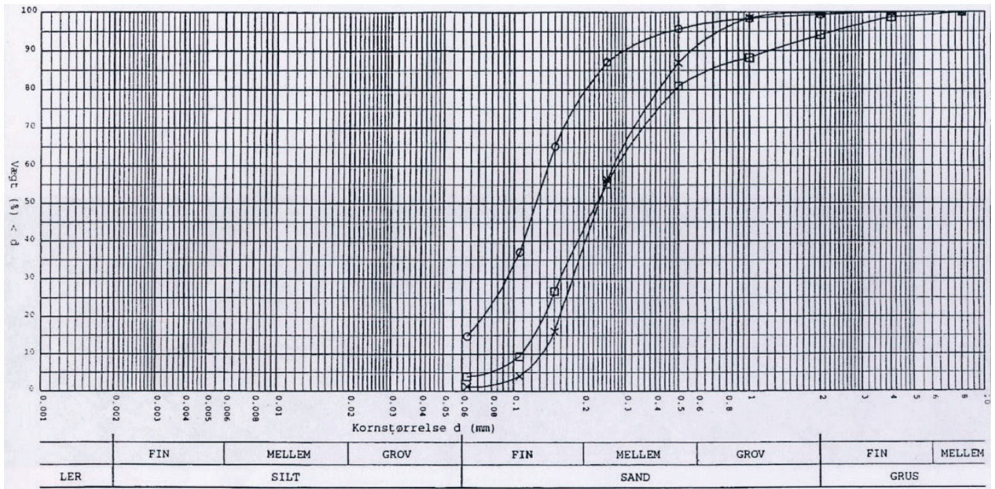
Figur 4 Kornkurve af sandprøver optaget i indsejlingen til Egå Marina i 1993.
