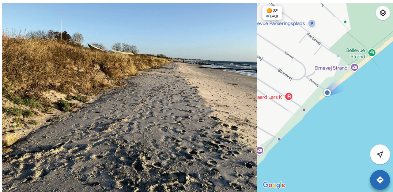
Foto 5 Kysten ud for Elmevej (set mod nord, se blå prik på kort til højre). Diget ses at være meget stejl som følge af erosion af digefoden.
