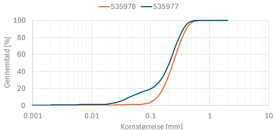
Figur 3 Kornkurver fra Egå Marinas indsejling. Prøver taget i november 2024.
