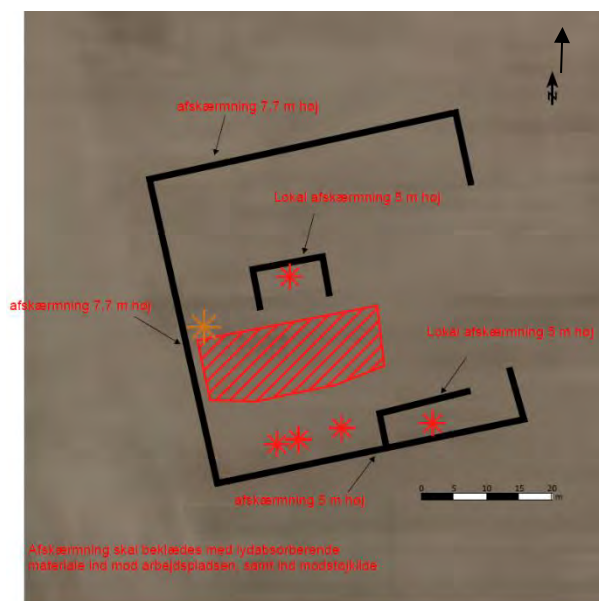
Figur 4: principtegning med placering af støjskærm ved Falster ved Lolland. Støjskærm fremgår som sort streg.
