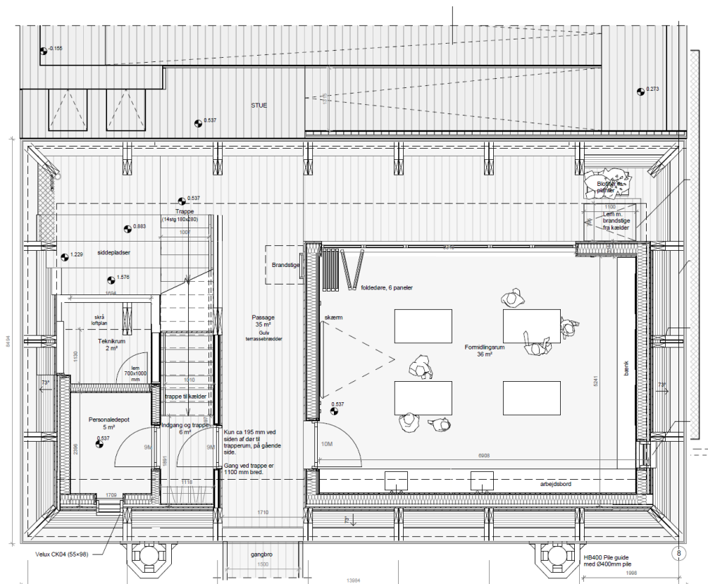
Formidlingspram inkl. del af læringsplatform – plantegning stue.
