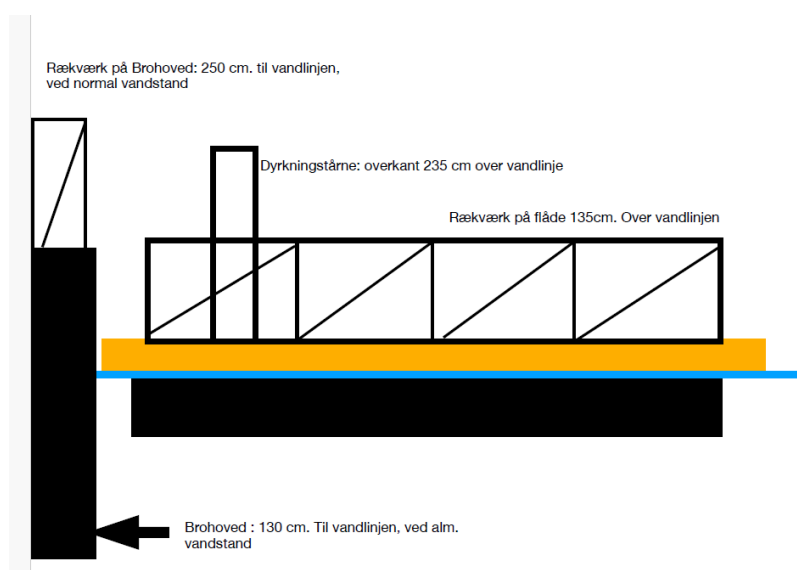
Figur 3: Tværsnit af platform og brohovedet
