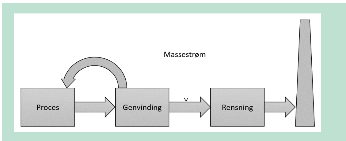
FIGUR 10. Sted, hvor massestrømmen bestemmes, hvis der sker genvinding af fx organiske opløsningsmidler fra spildgassen og genindvindingen er en integreret del af processen
