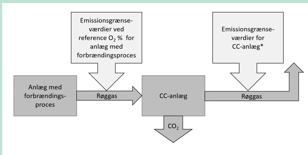
FIGUR 18. Illustration af, hvor emissionsgrænseværdier for hhv. anlæg med forbrændingsproces og CC-anlæg gælder. * For støv og NH 3 mv. fra CC-anlægget henvises til teksten over figuren.
