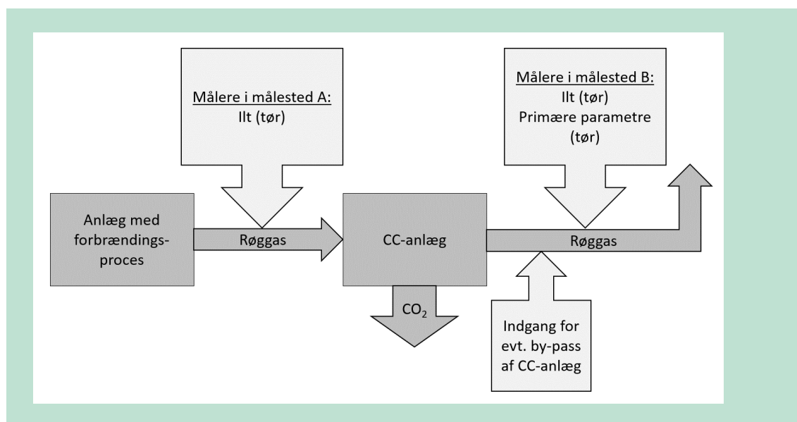
FIGUR 20. Målere og målesteder ved omregning af emissionskoncentrationer ud fra O 2 -målinger før og efter CC-anlæg. Primære parametre for anlæg med forbrændingsprocesser er NO x ,
