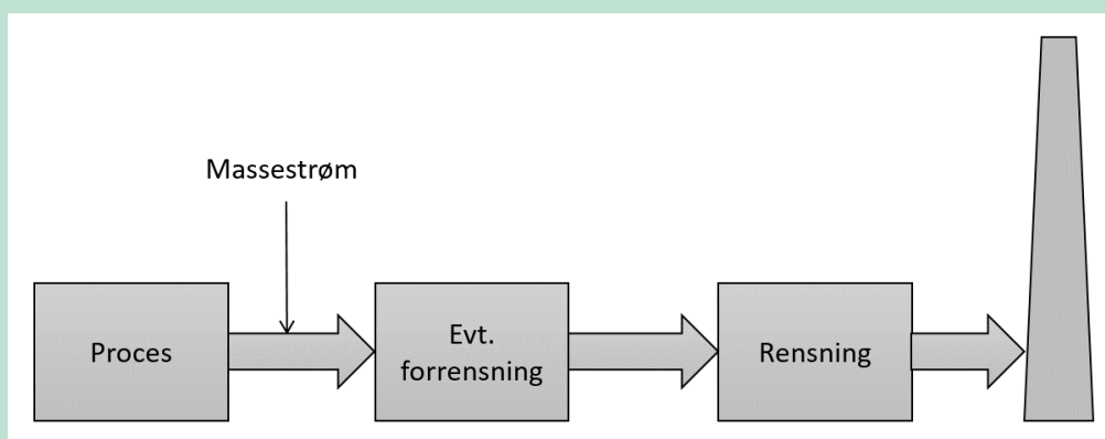
FIGUR 9. Sted, hvor massestrømmen bestemmes, hvis der er rensning. Forrensning kan fx være et eller flere forfiltre til det egentlige filter.
