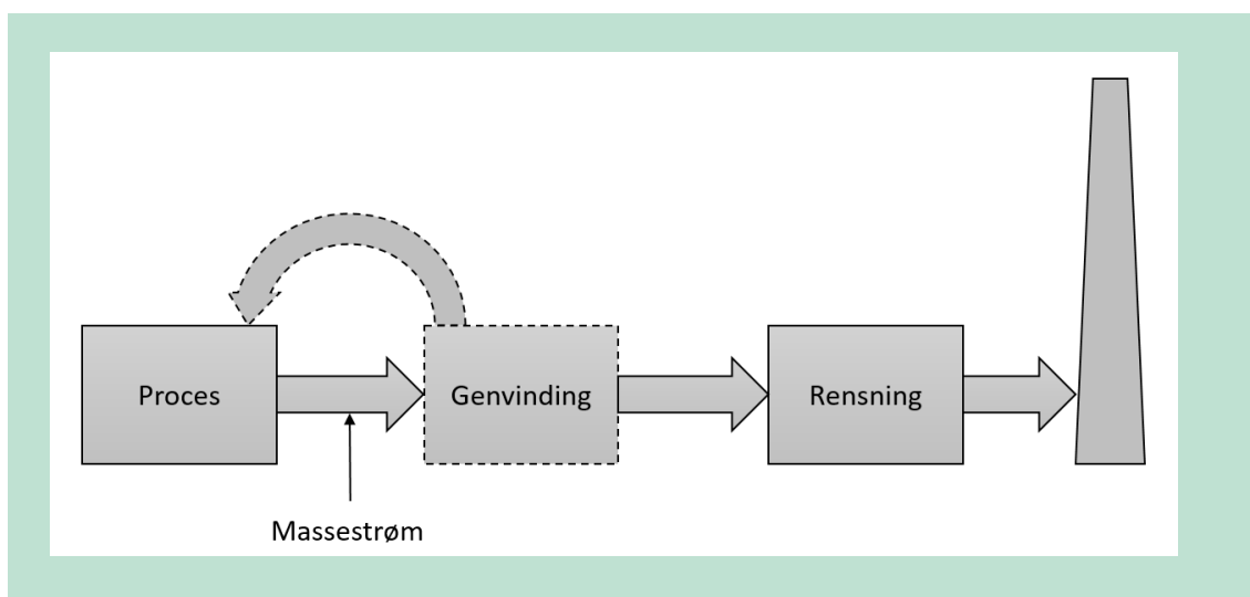
FIGUR 11. Sted, hvor massestrømmen bestemmes, hvis der periodevist sker genvinding af materialer fra spildgassen
