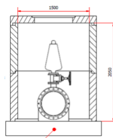
Figur 8: Principskitse af udluftningsbrønd
