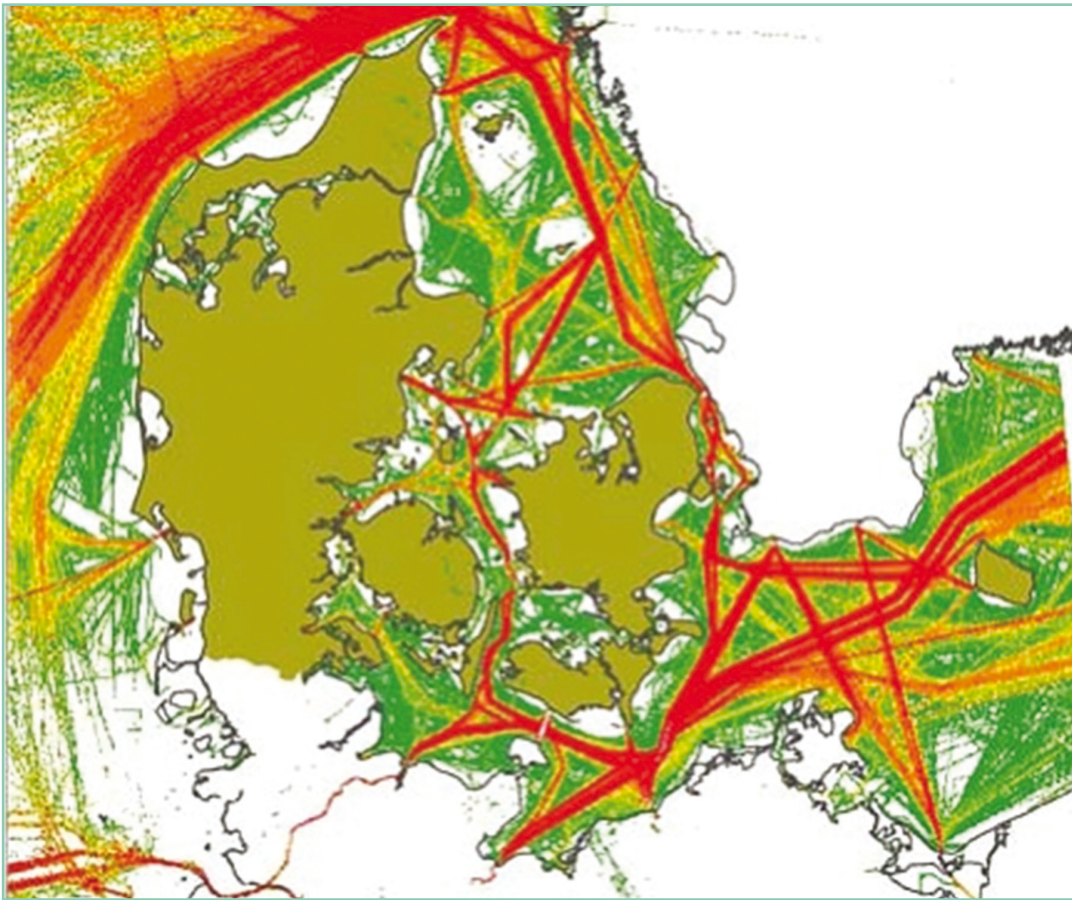
Figur 4 7 SO2-udslippet fra skibsfart gennem farvandene omkring Danmark i 2011. Kilde: Renere Skibsfart, Det Økologiske Råd, 2011
