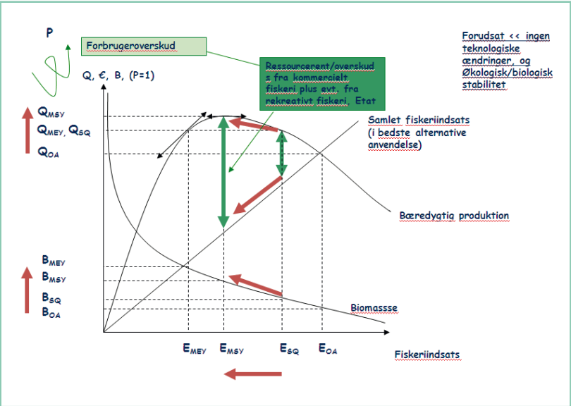
Figur 4.2 Præsentation af sammenhængen mellem biomasse, Bæredygtig produktion og Fiskeriindsats
