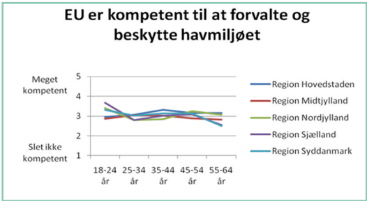
Figur 3 17 EU er kompetent til at forvalte og beskytte havmiljøet. Kilde: SDU, 2011
