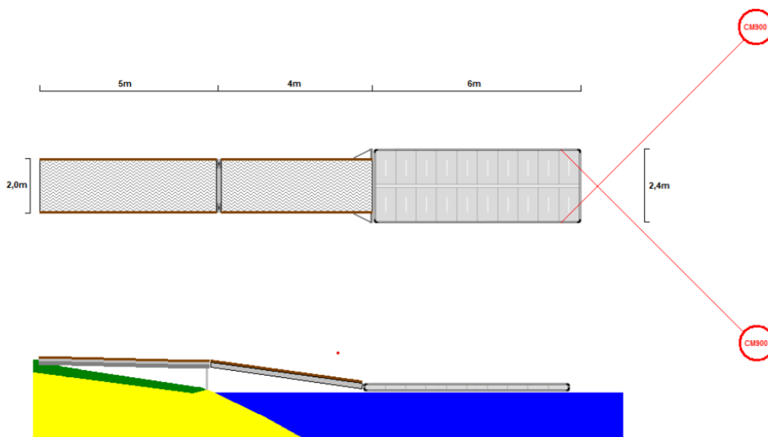
Fig. 2. Modtaget fra ansøger. Placering af flydebro på matriklen.
