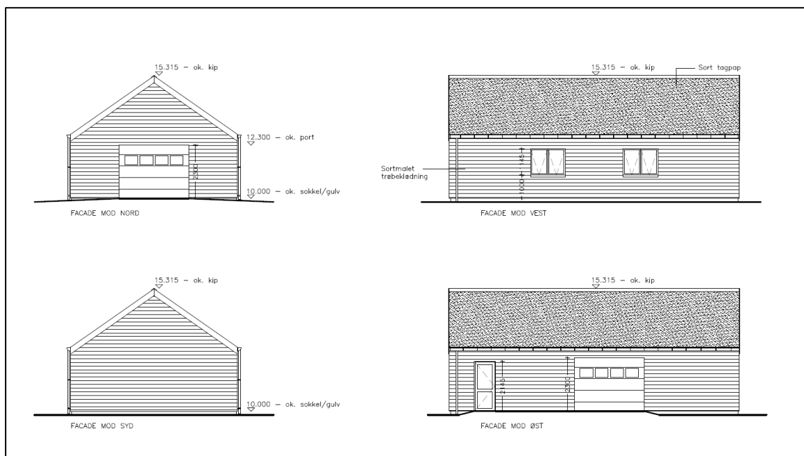
Skitse af den nye garage.
