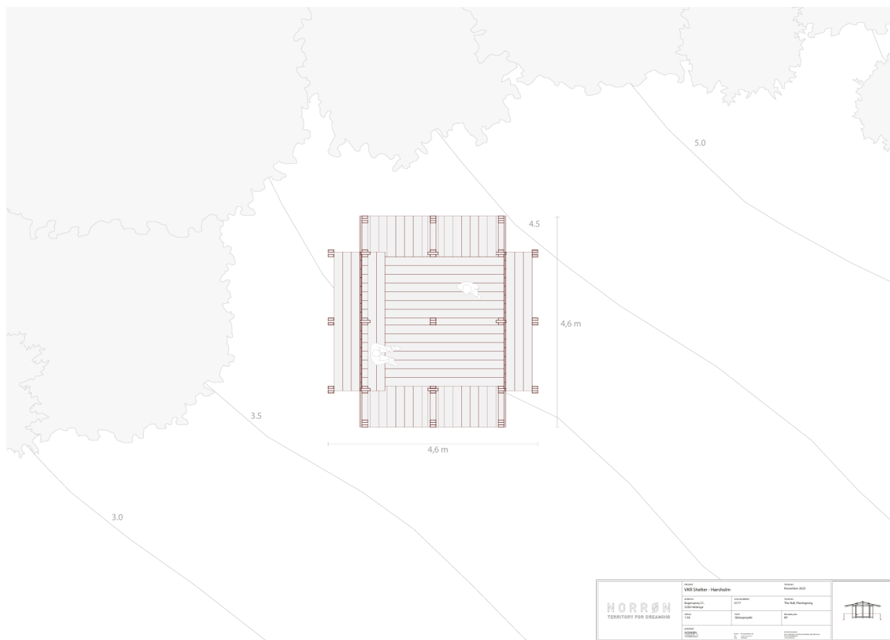
Fig. 6. Medsendt skitse af shelteren set oppefra.
