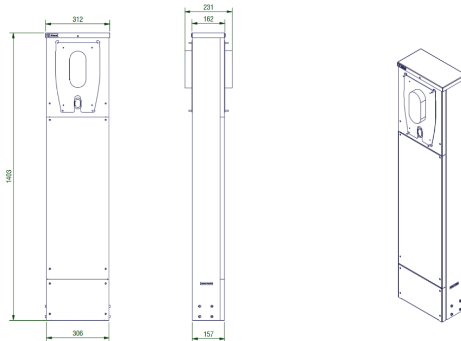
Fig. 4. Tilsendt fra ansøger. På figuren ses en illustration af ladestanderens mål.
