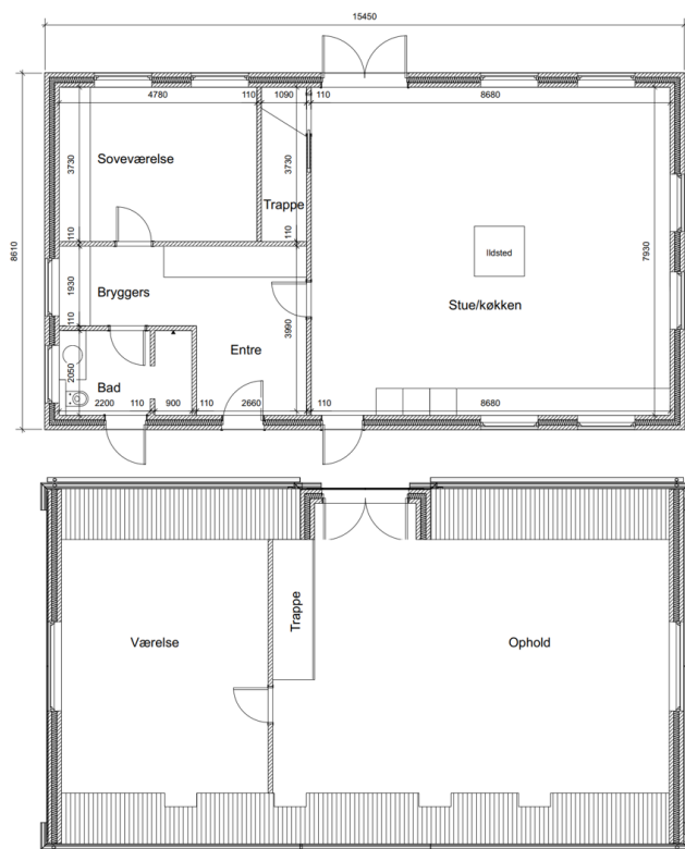
Fig. 4. Plantegning over henholdsvis stueplan og tagetage i det ansøgte hus.
