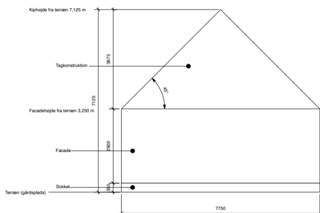
Fig. 2. Tegning indsendt af ansøger som viser taghøjde- og hældning.
