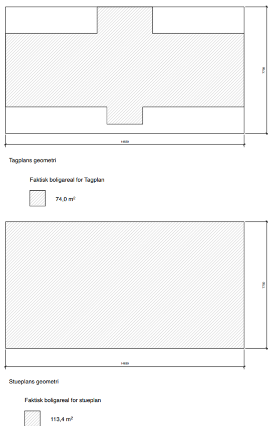
Fig. 3. Tegning indsendt af ansøger, hvorpå boligarealet i stue- og tagetage i det eksisterende hus er markeret.
