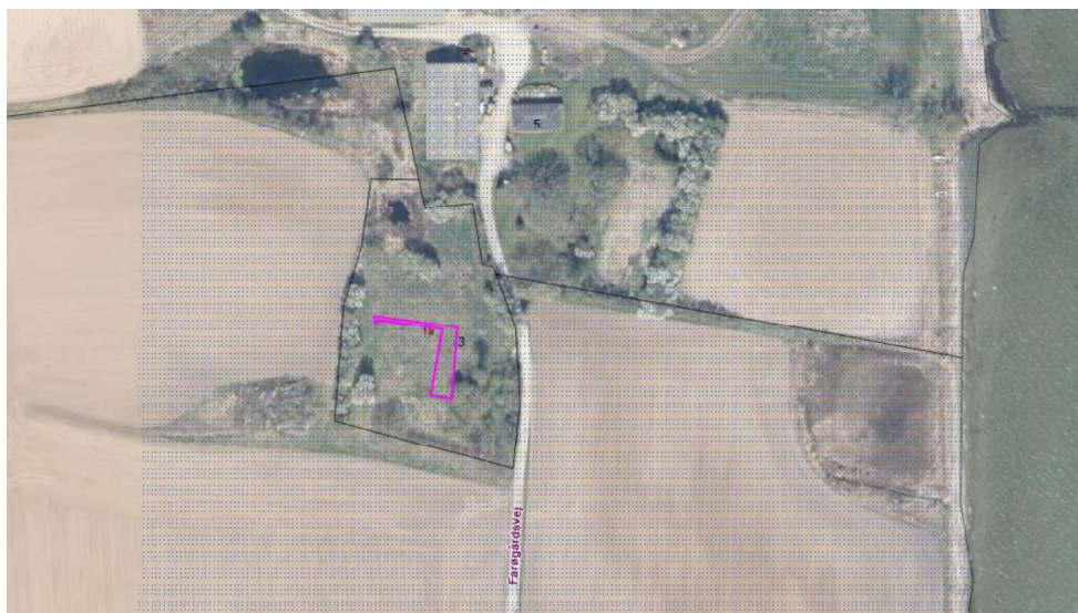
Fig. 2 Beskrivelse af placering af jordvarmeslanger. Fra ansøgningsmaterialet.
