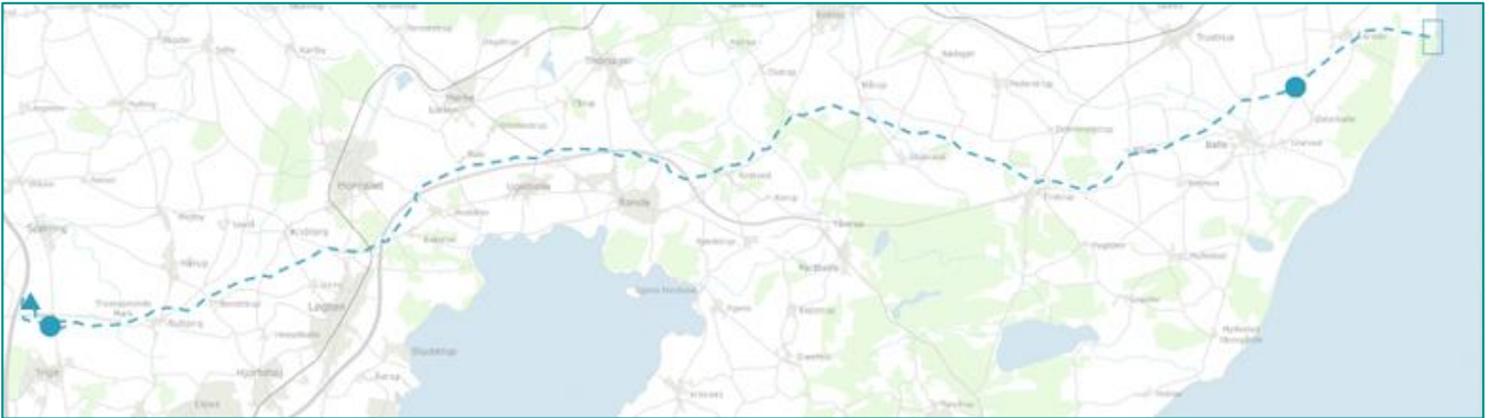
Figur 1-2 Placering af projektet Mere Havvind 2030 Kattegat Havvindmøllepark til Trige, hvor firkanten angiver placering af ilandføringspunktet, cirklerne angiver placering af koncessionsvindens anlæg (øst: kompensationsstation, vest: koblingsstation) og trekanten angiver placering af eksisterende højspændingsstation ved Trige. Den stiplede linje angiver placering af landkabeltracé.
