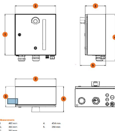
Fig. 4. Tilsendt fra ansøger. Billede og skitse af ansøgte control unit til ladestanderen.
