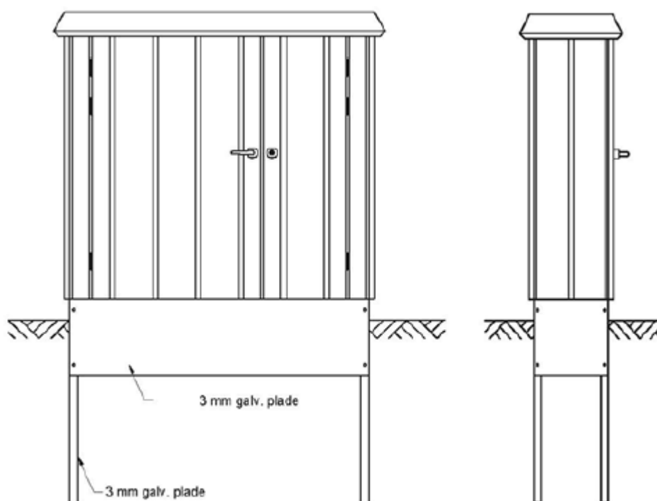
Fig. 5. Tilsendt fra ansøger. Skitse af ansøgte eltavle.
