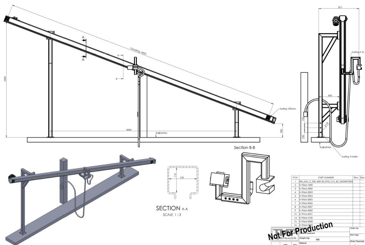
Fig. 3. Tilsendt fra ansøger. Skitser af den ansøgte ladestander til færgen med mål.
