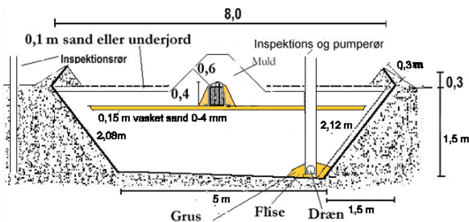
Fig. 4. Målskitse færdigt bassin (alle mål i m). Fra ansøgningsmaterialet.
