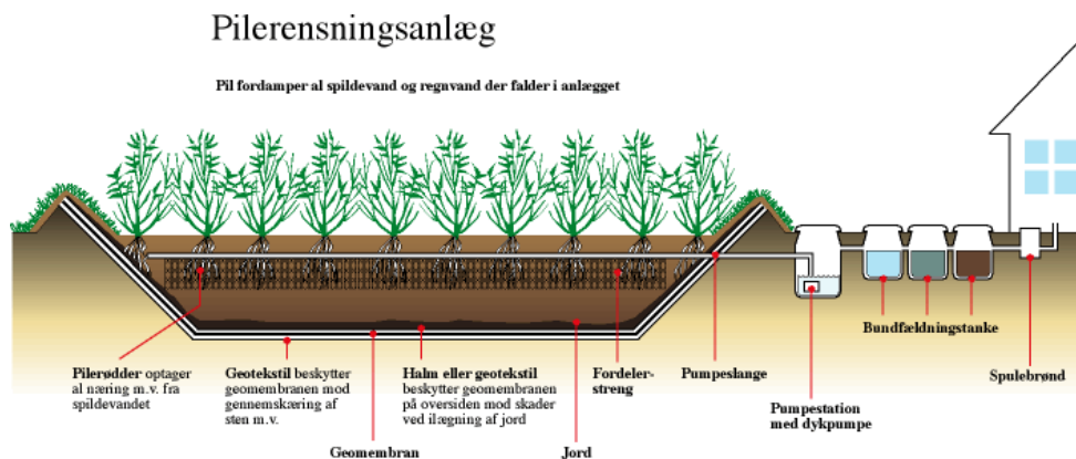
Fig. 5. Illustration af pilerenseanlægget. Fra ansøgningsmaterialet.
