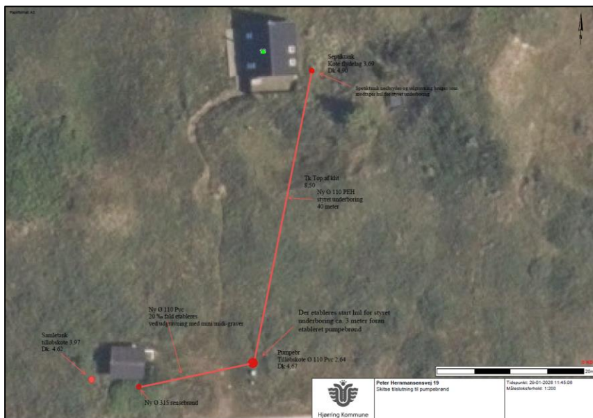
Fig.2. Tilsendt af ansøger. Oversigtstegning over rørføringer og placering af brønde.
