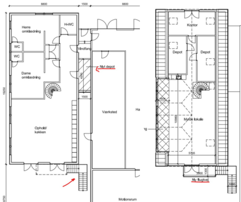
Stueplan: depotrum og trappe
