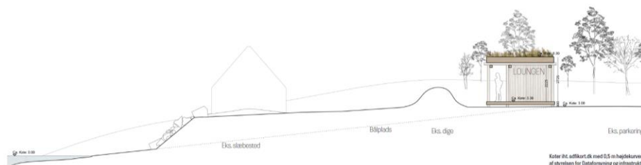
Fig. 5. Tilsendt fra ansøger. På tegningen kan man se, hvor de forskellige anlæg på matriklen (madpakkehus, bålsted, dige, bygning, parkeringsplads) er placeret i forhold til kysten.
