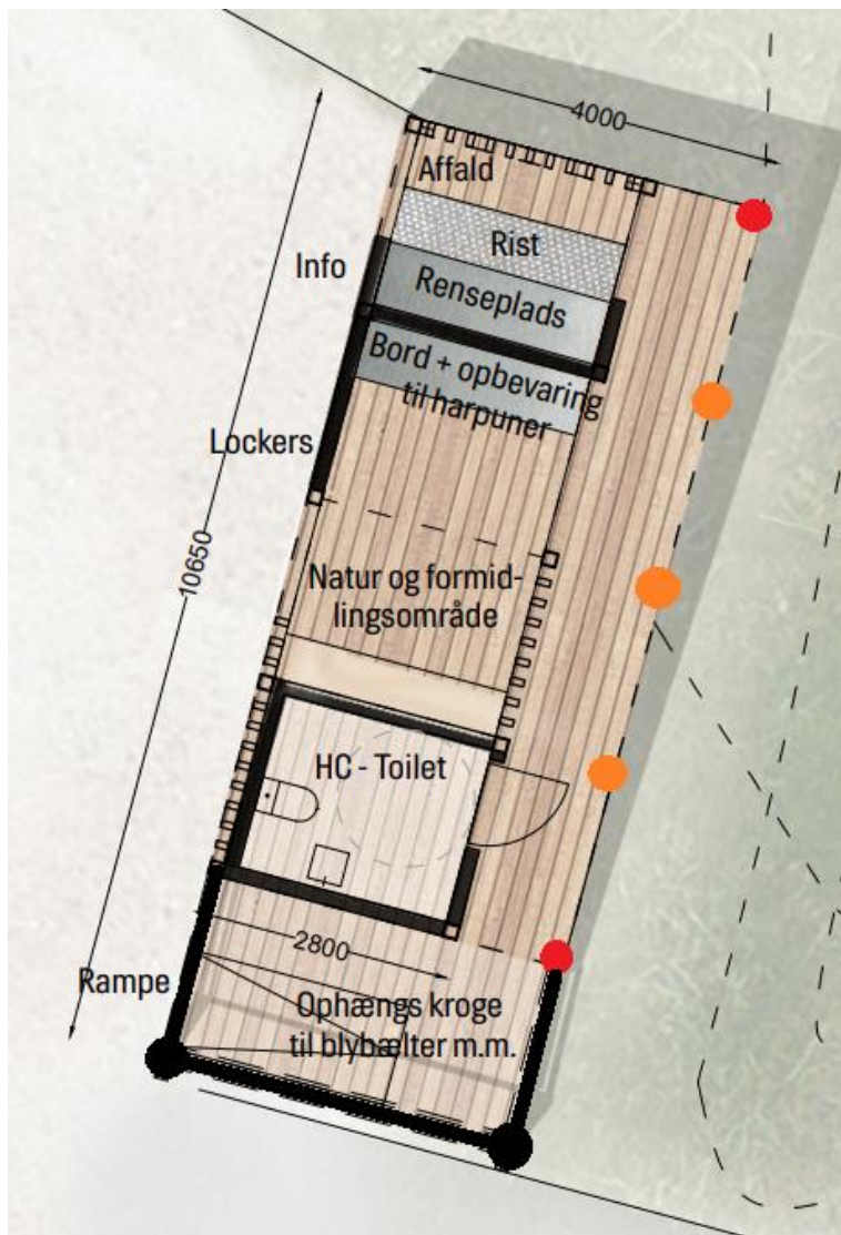
Fig. 8. Tilsendt fra ansøger. På figuren ses en tilrettet tegning af den ansøgte formidlingsbygning. Søjler og bjælker markeret med sort fjernes. Søjler markeret med orange fjernes. Søjler markeret med rød bibeholdes.
