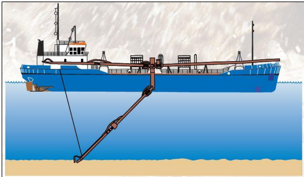
Figur 4-3. Skitse af metoden bag slæbesugning (Kystdirektoratet, 2012).
