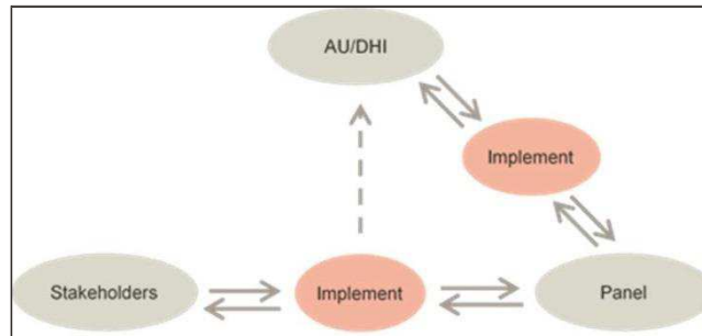
Figur 1. Kommunikationsmodel
