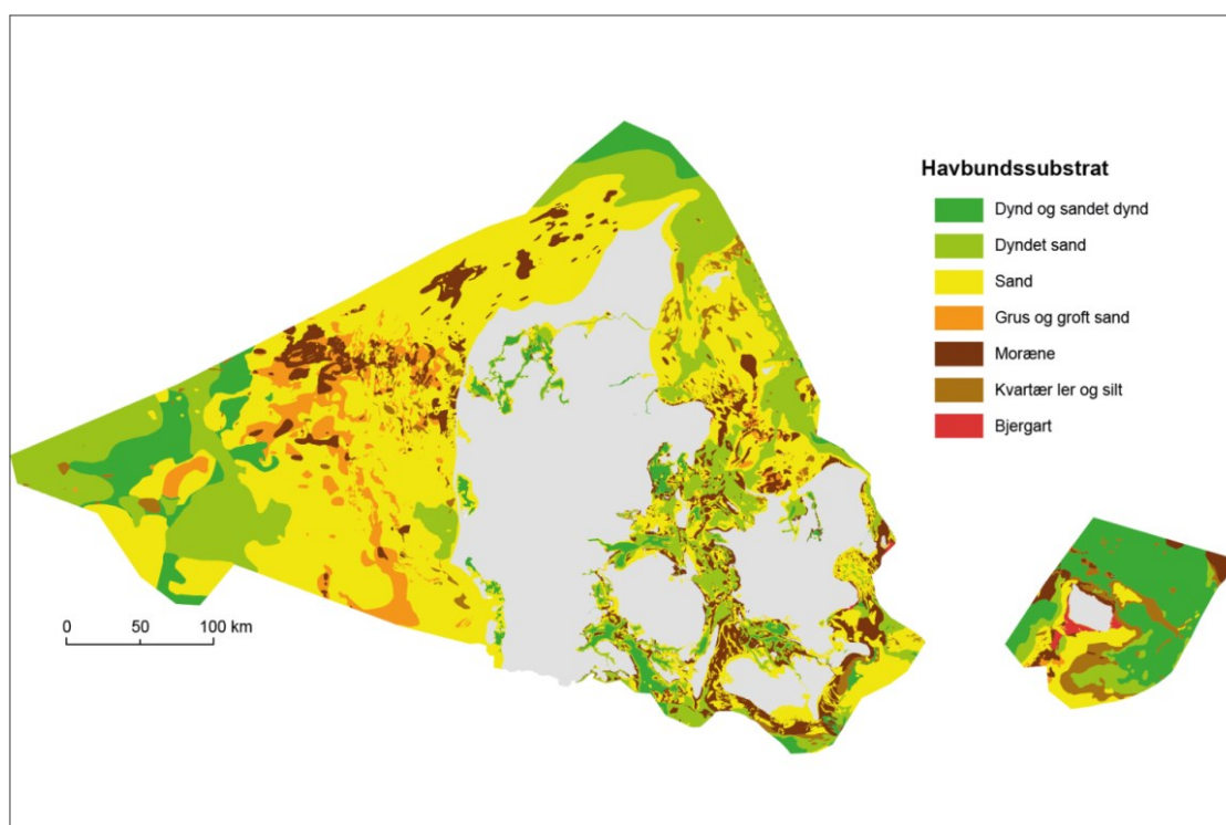
Figur 6.2: Havbundssubstrater [3].
