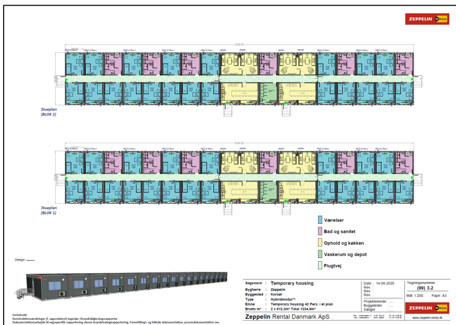
Fig. 3 Tilsendt af ansøger. Konstruktionstegning af beboelsesfaciliteterne.
