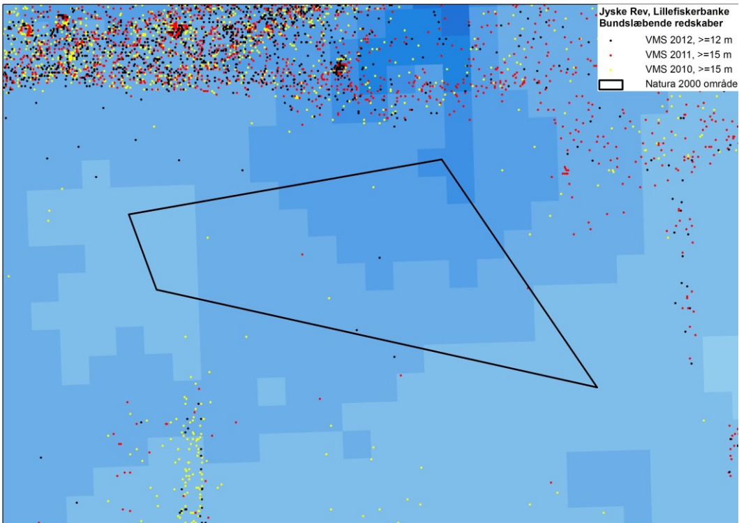
VMS positioner for fiskerifartøjer over 12 m, der fiskede med bundsløbende redskaber. Kort udarbejdet af DTU-Aqua.
