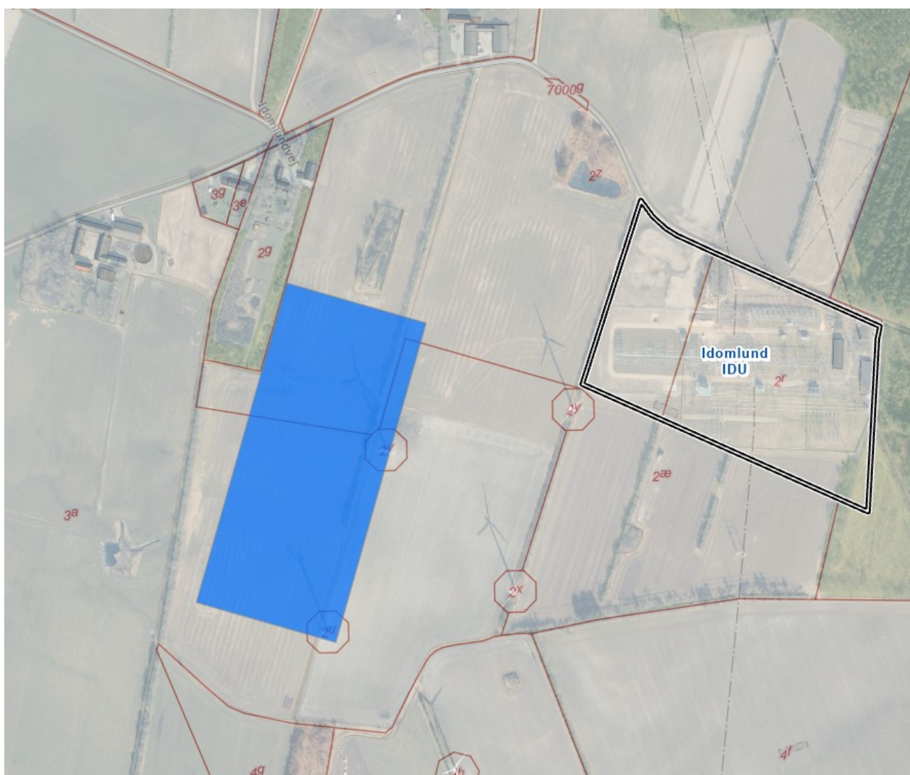
Figur 4-4. Den nye koblingsstation placeres i Holstebro kommune vest for den eksisterende station Idomlund og tilkobles denne. Arealet til stationen udgør ca. 7,2 ha (400x180m).
