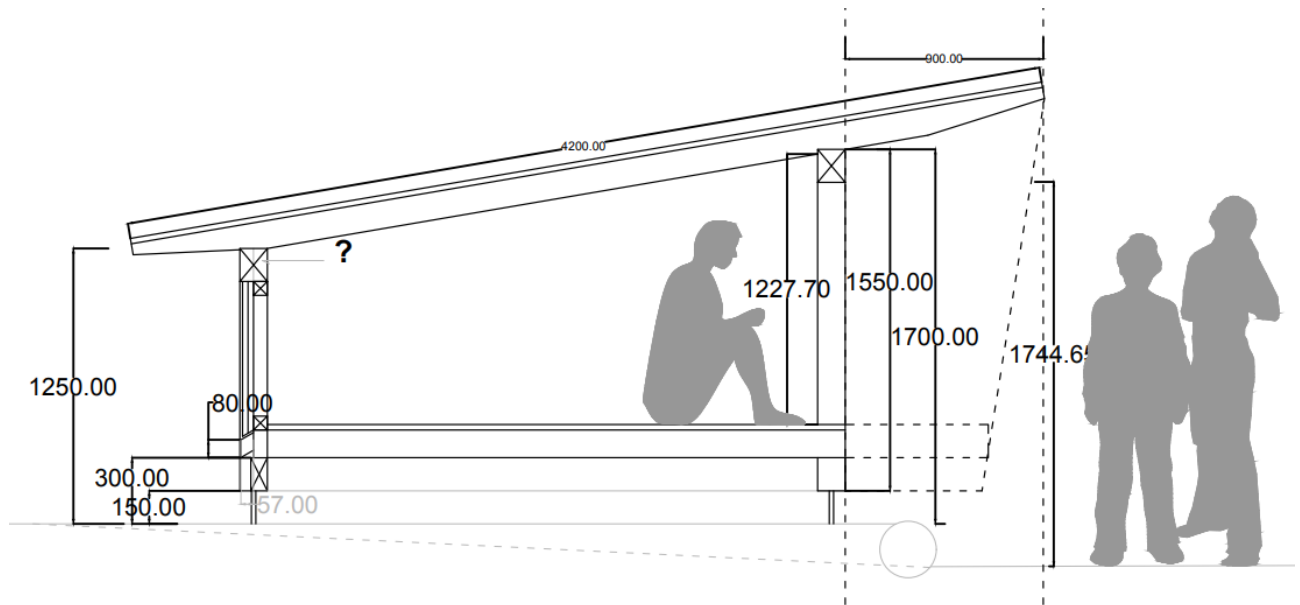
Fig. 2. Illustration af sheltertypen, der ønskes opført på ejendommen.
