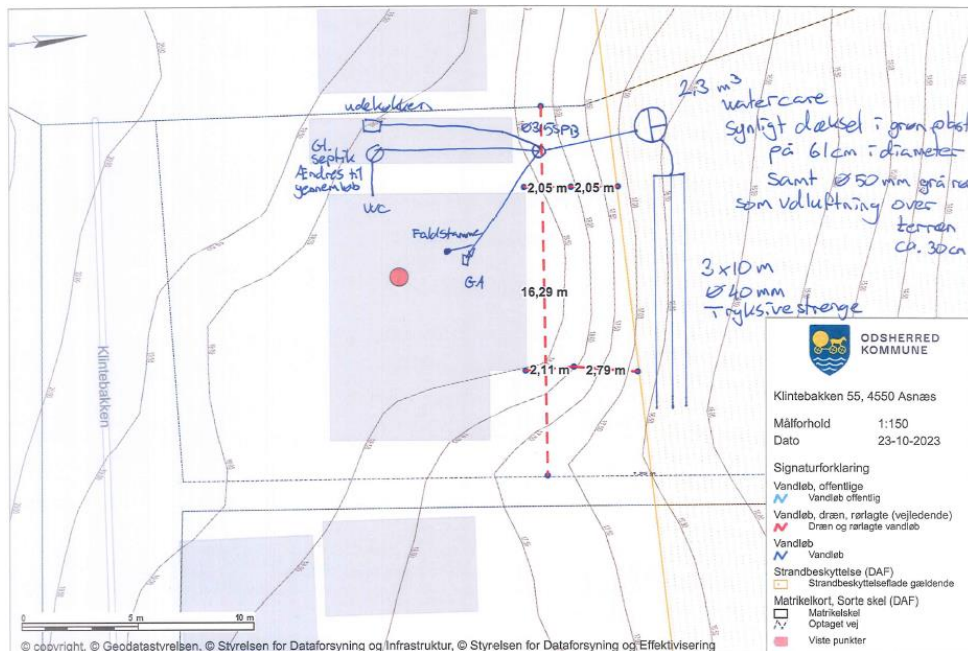
Figur 3. Skitse, fremsendt af ansøger. Anlægget består af en trekammer tank med dæksel Ø 61 cm i niveau med terræn, 3 nedgravede tryksivestrenge på hver 10 m, samt et udluftningsrør Ø 5 cm, der rager ca. 30 cm op over terræn.
