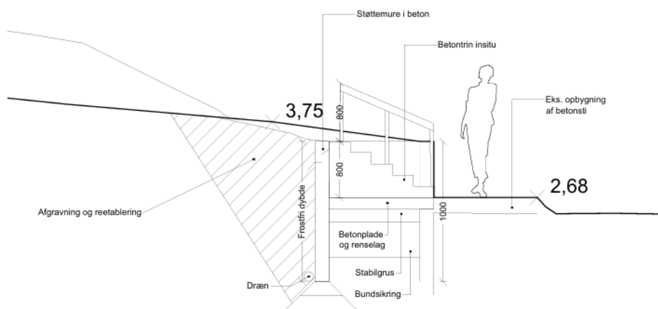
Snit E: Forbindelse fra eksisterende støttemur til strand med trappe med 5 trin 1:50
