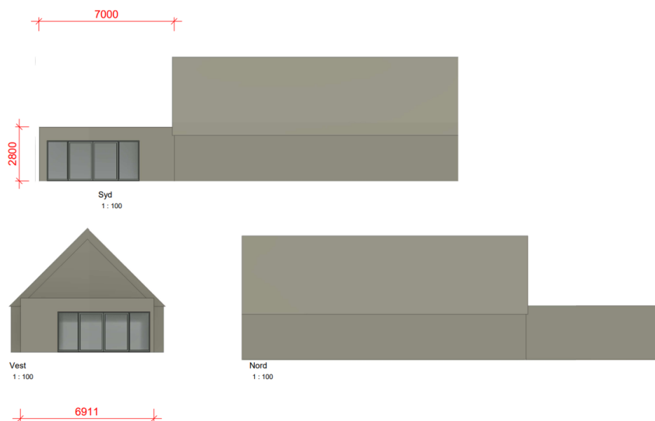
Fig. 3. Facadetegninger af den ansøgte udestue indsendt af ansøger.
