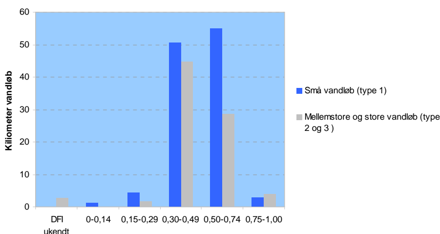
Figur 2.3.5. Den fysiske tilstand i små og mellemstore/store, åbne vandløb i Hovedvandopland Øresund, hvor denne er målt eller modelberegnet (i alt 196 km vandløb). Tilstanden er beskrevet ud fra normaliserede værdier af Dansk Fysisk Indeks. Rørlagte strækninger indgår ikke i opgørelsen. Data er opgjort i 2009/2010 og afgrænsning er opgjort i 2013.
