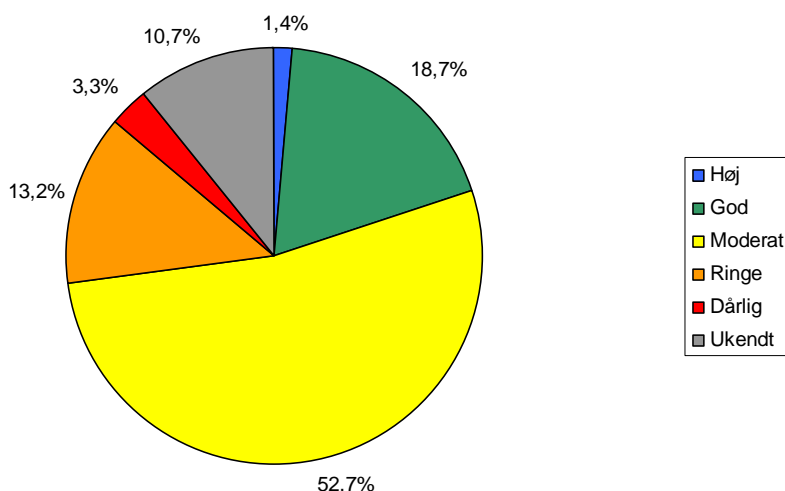
Figur 2.3.4. Økologisk tilstand eller økologisk potentiale i vandløb i Hovedvandopland Øresund, angivet som andelen af den samlede vandløbslængde (opgjort i 2009/2010).. Rørlagte strækninger er medregnet som ukendt tilstand.
