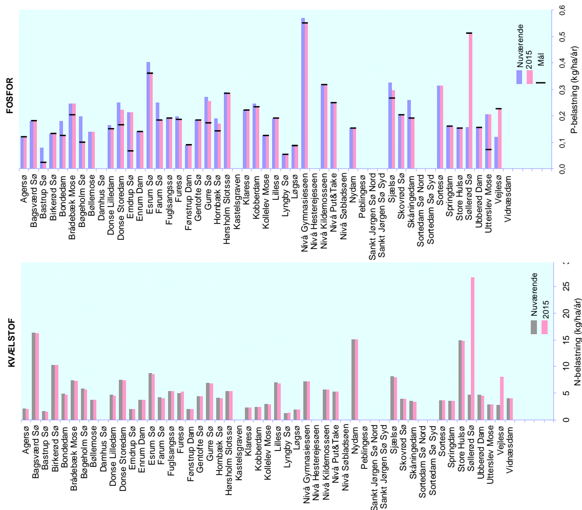
Figur 2.4.1. Den arealspecifikke kvælstof- og fosforbelastning af søerne i oplandet, dels under beregnet pba data opgjort i 2009/2010 belastningsforhold og dels den fremskrevne belastning (baseline 2015). Fosforbelastningen ved målopfyldelse fremgår tillige
