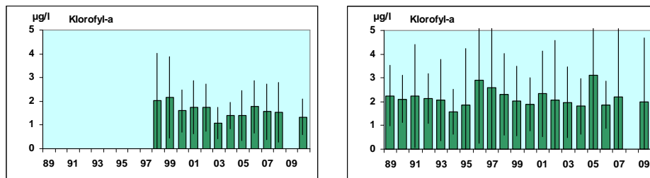
Figur 2.3.7. Koncentrationer af total-N, total-P og klorofyl opgjort som årsmidler fra 1989 til 2009 for overfladevandet ved Gilleleje (FRB1939) og Nivå Bugt (FRB1877).
