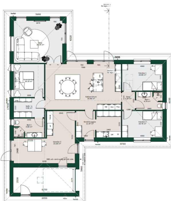
Fig. 3. Tilsendt fra ansøger. På figuren ses en plantegning over det ansøgte hus.
