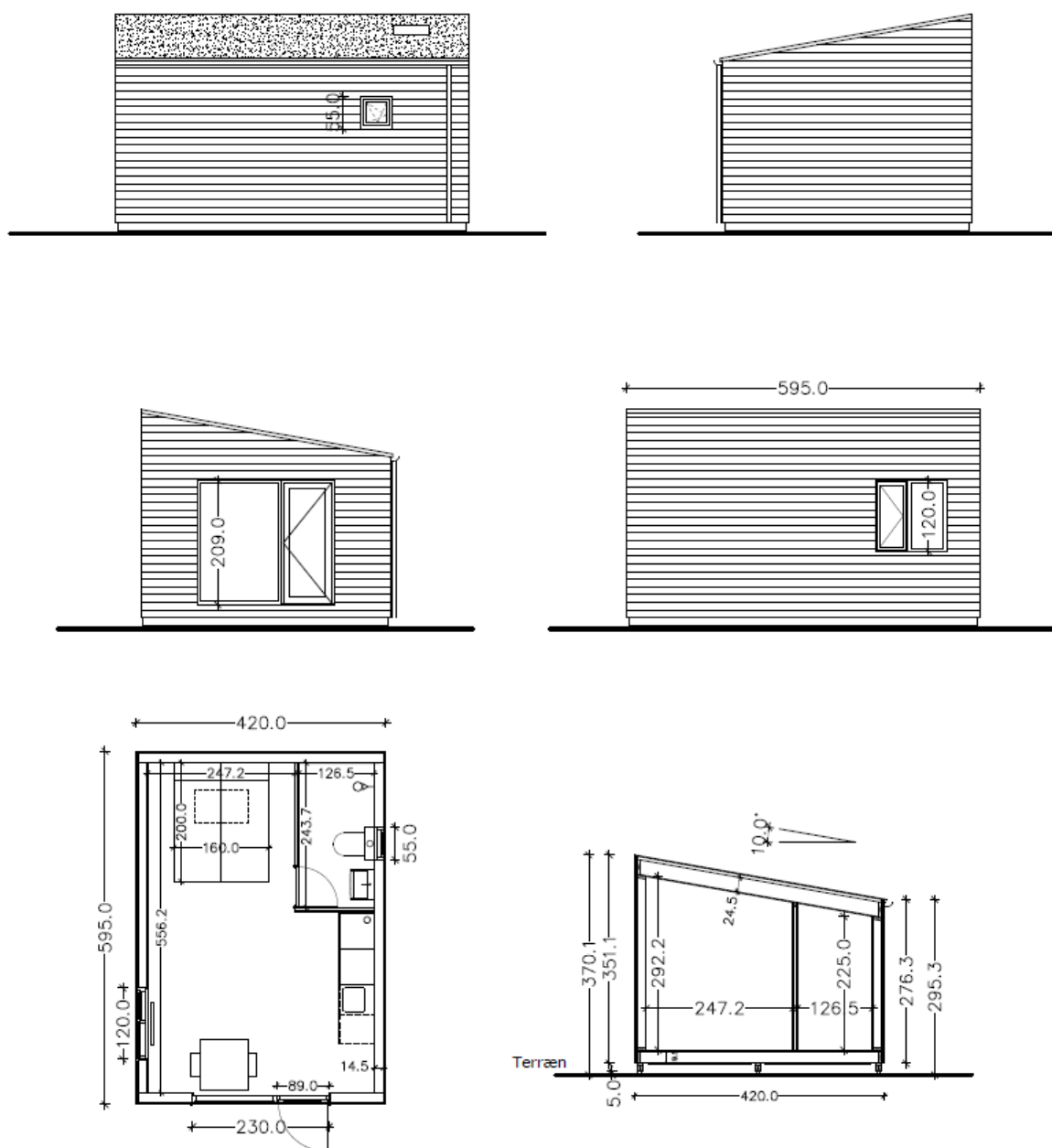
Fig. 4. Tilsendt fra ansøger. På figuren ses tegninger af en campinghytte på 25 m 2 .
