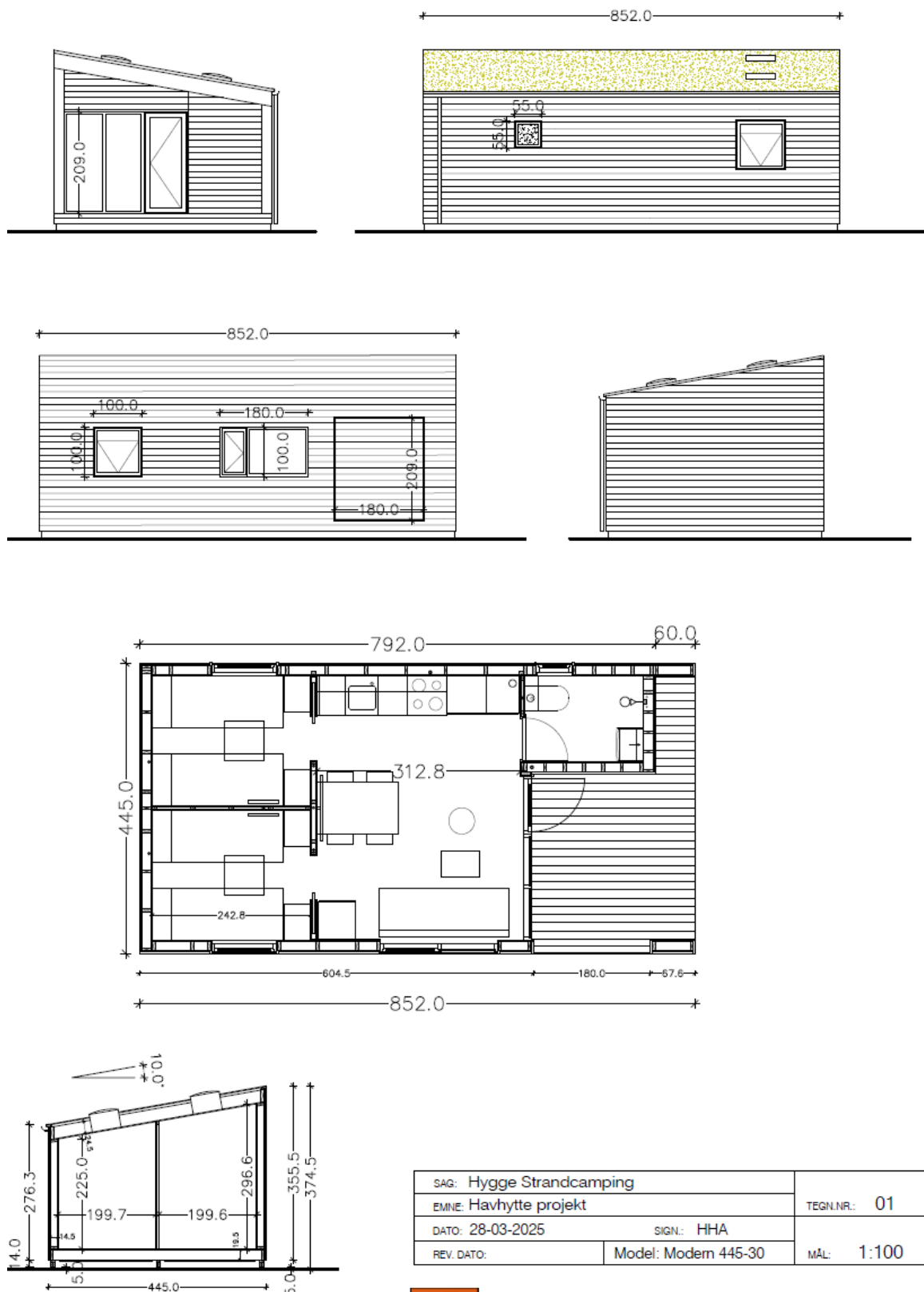
Fig. 5. Tilsendt fra ansøger. På figuren ses tegninger af en campinghytte på 30 m 2 .
