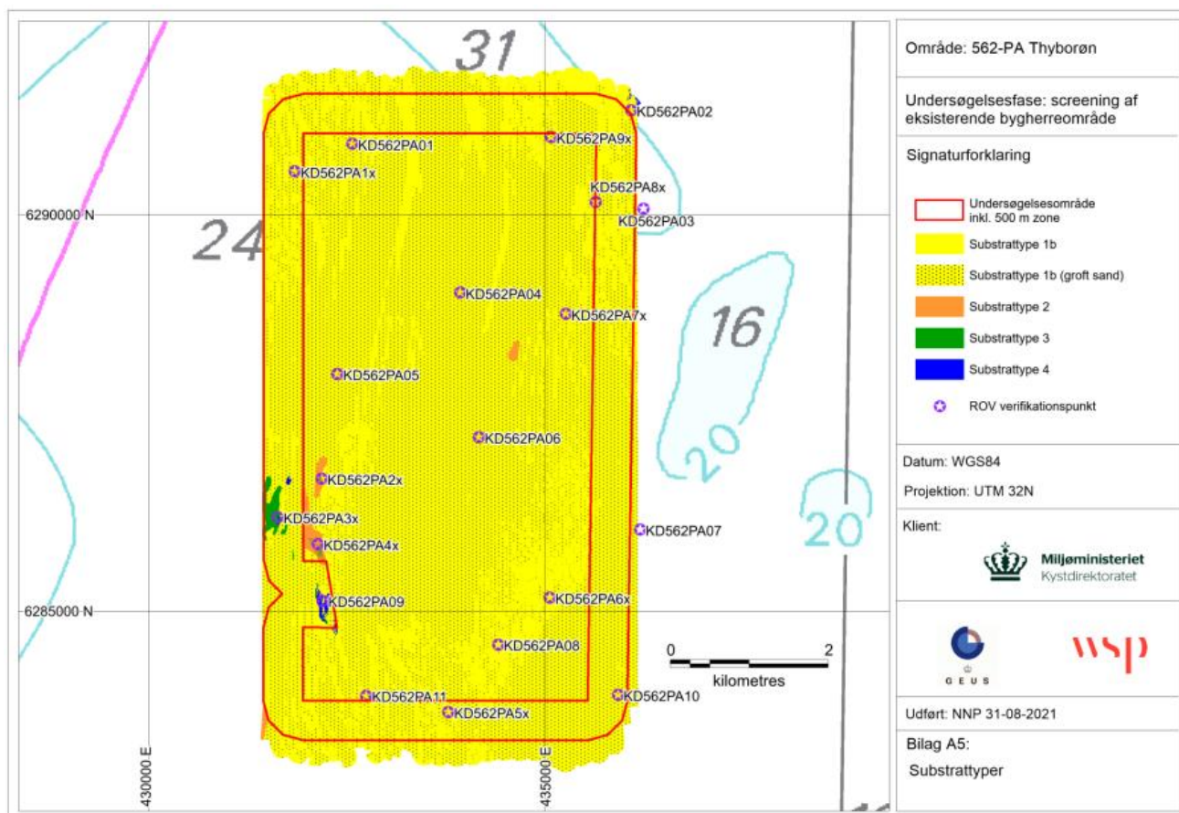
Figur 7-3. Substrattypekort for efterforskningsområdet 562-PA Thyborøn, der viser fordelingen af de tolkede substrat typer. Desuden er angivet lokaliteter for de gennemførte ROV stationer (GEUS, 2021).
