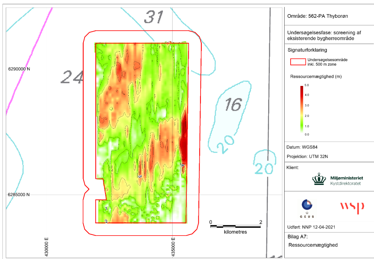
Figur 7-4. Kortlagt tykkelse af sandressourcen inden for område 562-PA Thyborøn (GEUS, 2021a).
