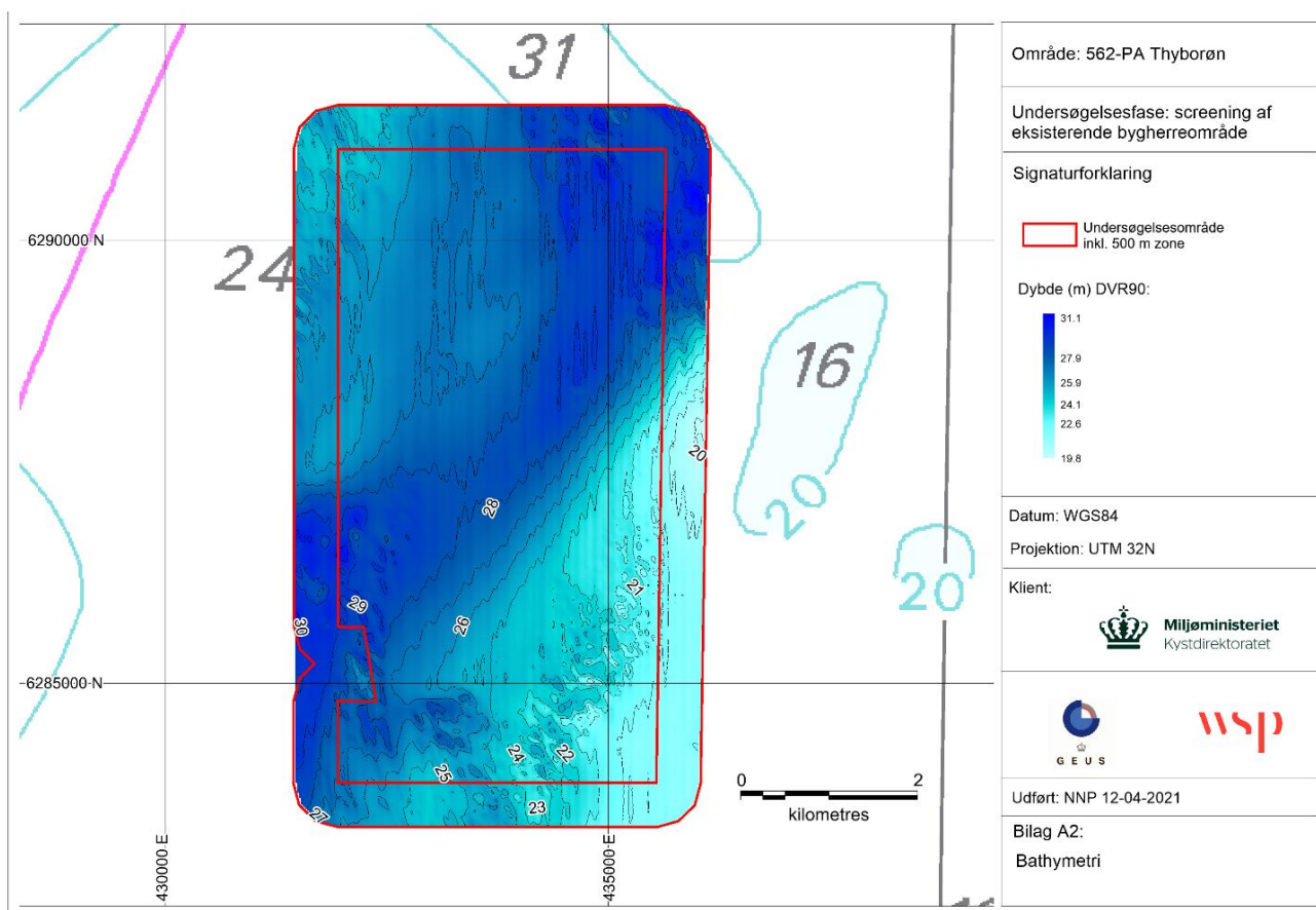
Figur 9-1. Dybdekort (bathymetrisk kort) for ansøgningsområdet og med tilhørende påvirkningszone med angivelse af 1 m konturlinjer i forhold til DVR90. Kilde: (GEUS, 2021).
