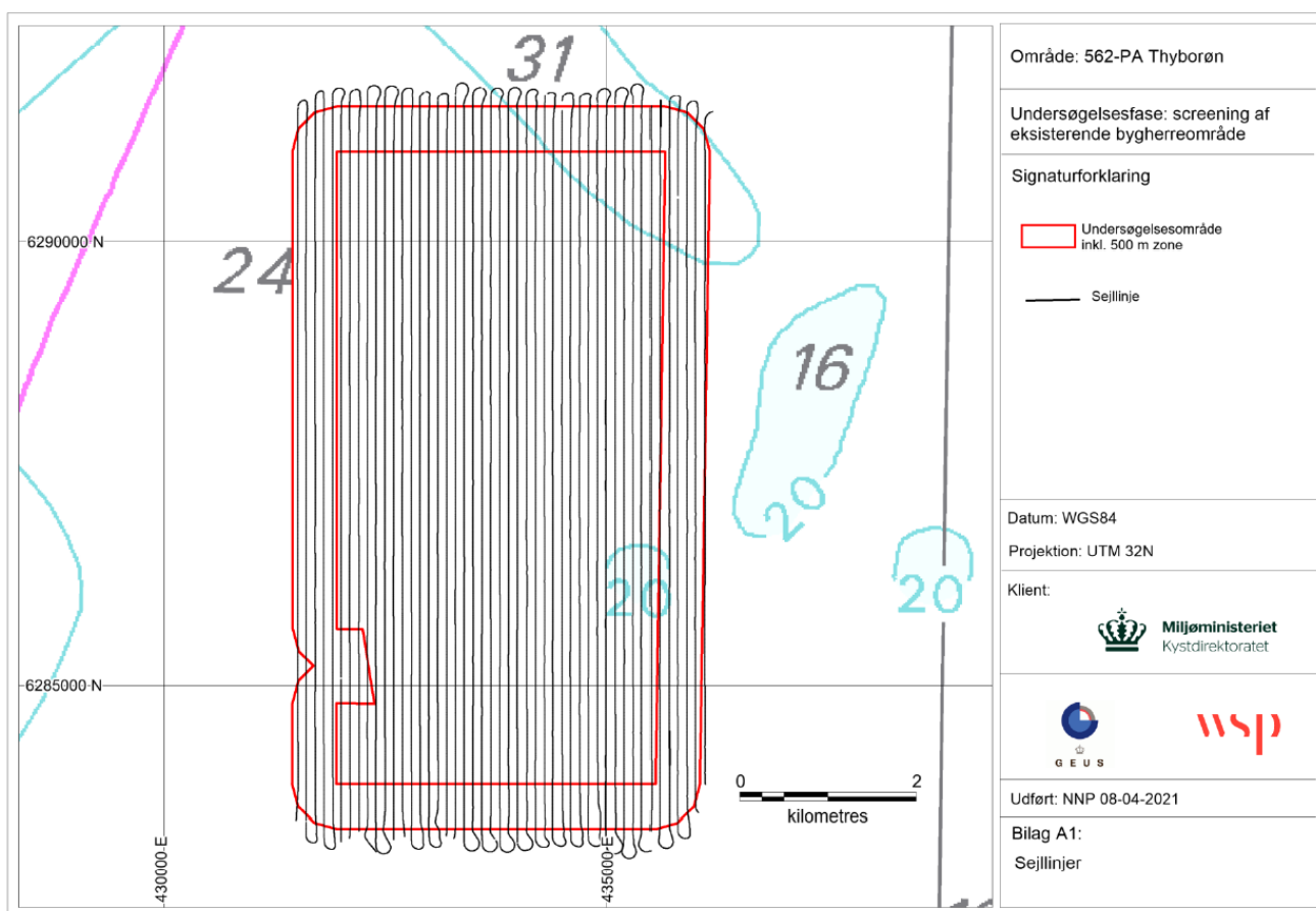
Figur 7-1. Oversigt over sejlede geofysiske surveylinier i bygherreområde 562-PA Thyborøn og tilhørende 500 m påvirkningszone (GEUS, 2021).
