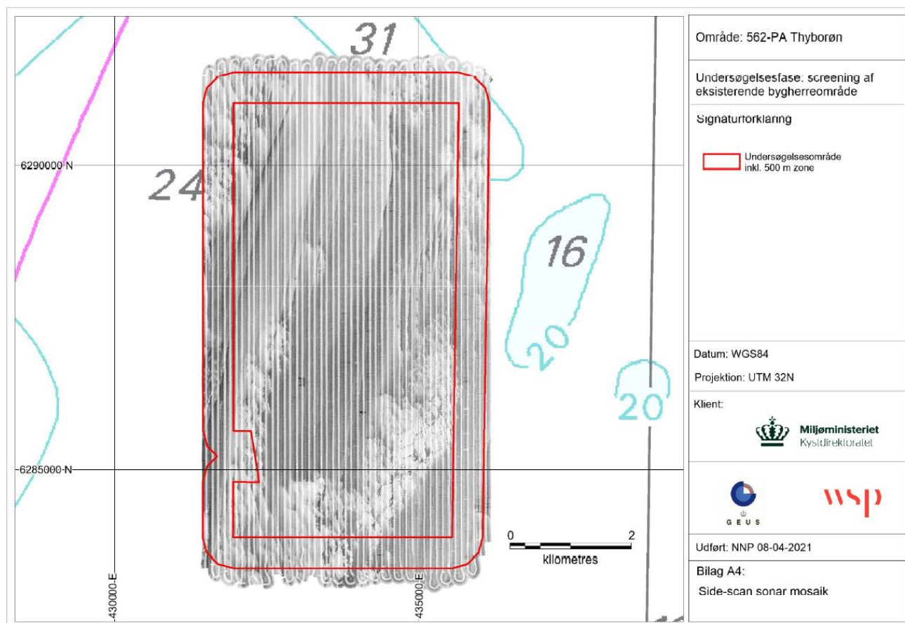
Figur 7-2. Side Scan Sonar mosaik for bygherreområde 562-PA og tilhørende 500 m påvirkningszone (GEUS, 2021).
