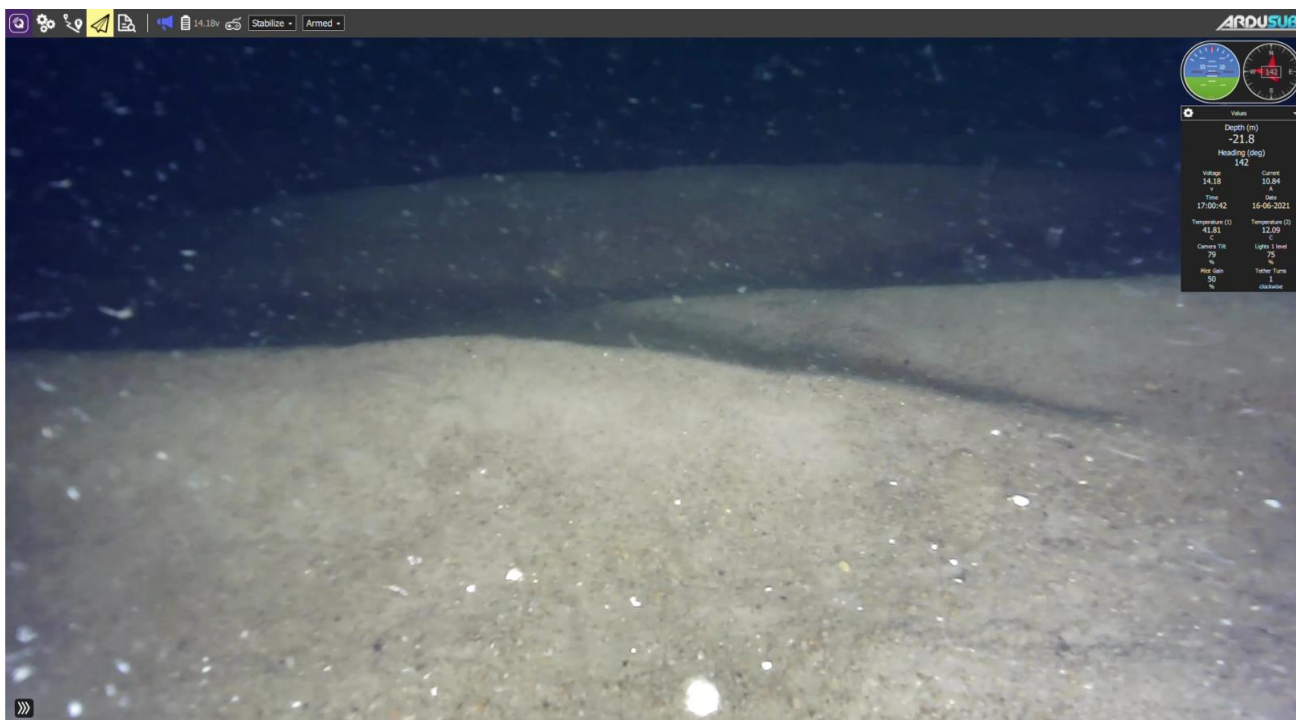
Figur 9-9. Dynamisk sandbund med kraftige bølge- og/eller strømribber. Eksemplet er fra den sydøstlige del af påvirkningszonen ved ROV station 10.
