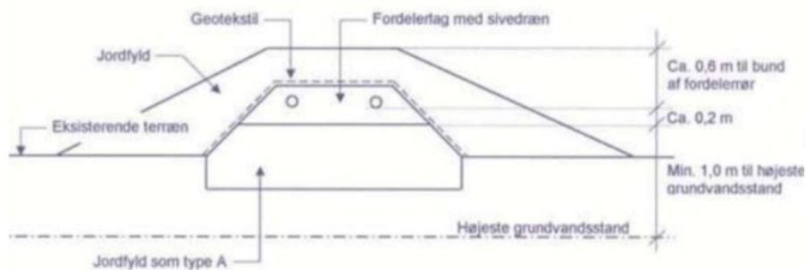
Snittegning med eksempel på anlæggets opbygning
