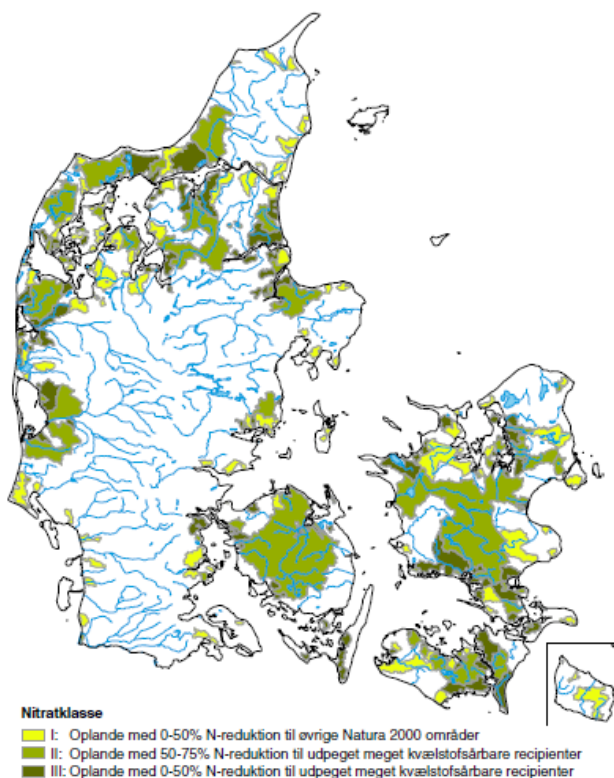
Figur 1. Nitratklassekort (DCE, 2007).
