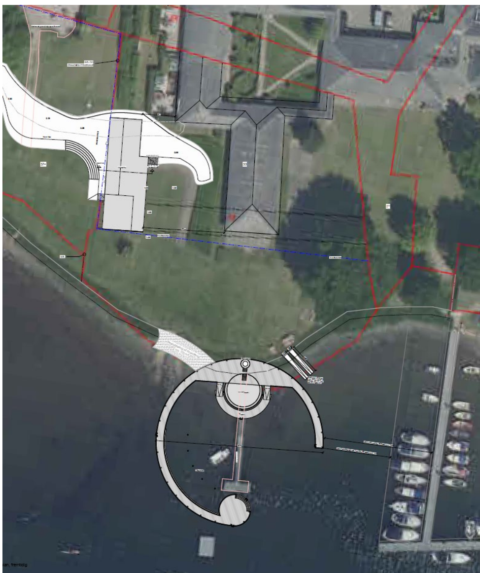
Figur 1. Situationsplan over projektet som helhed. Nærværende ansøgninger omhandler etableringen af slæbepladsen øst for brodækket.
