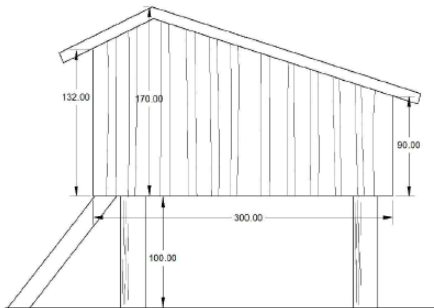
Fig. 3. Tegninger af den ansøgte shelter fra tilsendte landzonetilladelse.
