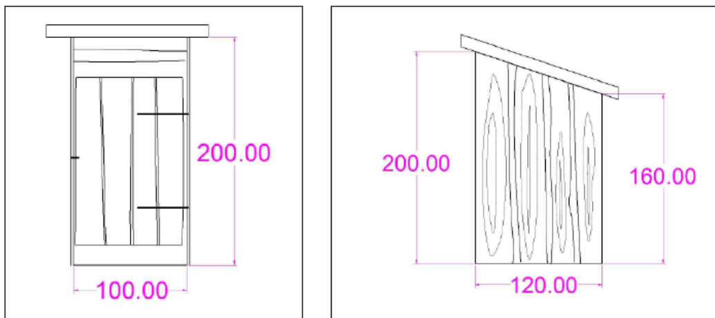
Fig. 5. Tegninger af det ansøgte muldtoilet fra tilsendte landzonetilladelse.
