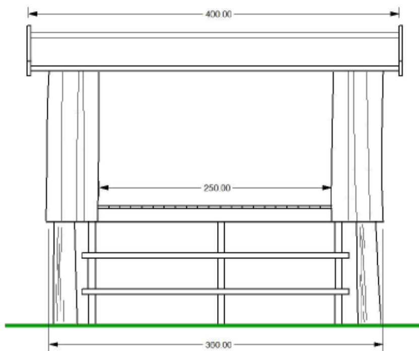
Fig. 4. Tegninger af den ansøgte shelter fra tilsendte landzonetilladelse.
