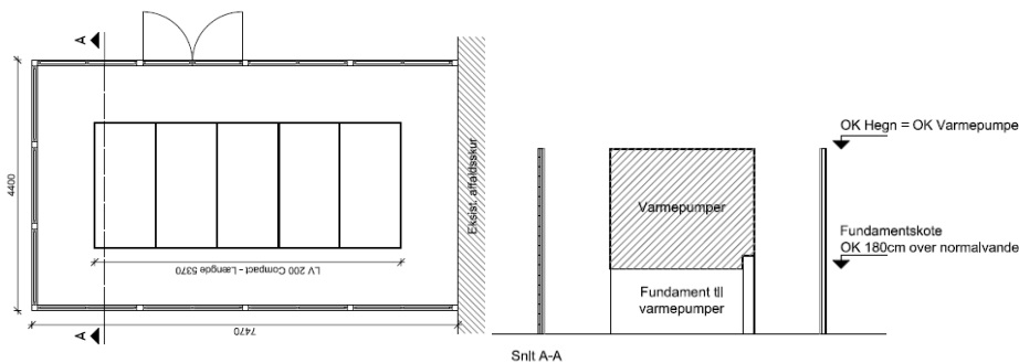
Gård med varmepumper ved bygning B12 – placering vist med rød under
