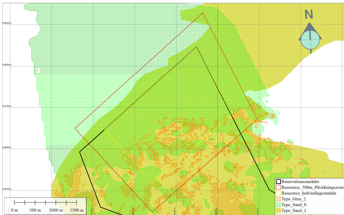
Figur 9 Oversigt over overfladesedimentkort udarbejdet af GEUS. Data tilgængelige i Marta-databasen
