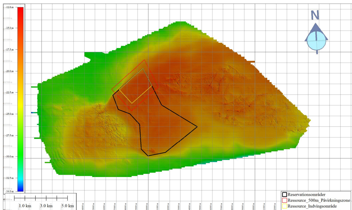
Figur 1 Bathymetrisk oversigt over hele Kriegers Flak området. Sort areal viser område udlagt til mulige reservationsområder. Gult areal viser efterforskningsområde ansøgt af By & Havn med henblik på senere indvindingssansøgning. Rød viser 500m påvirkningsområde for potentielt indvindingssområde
