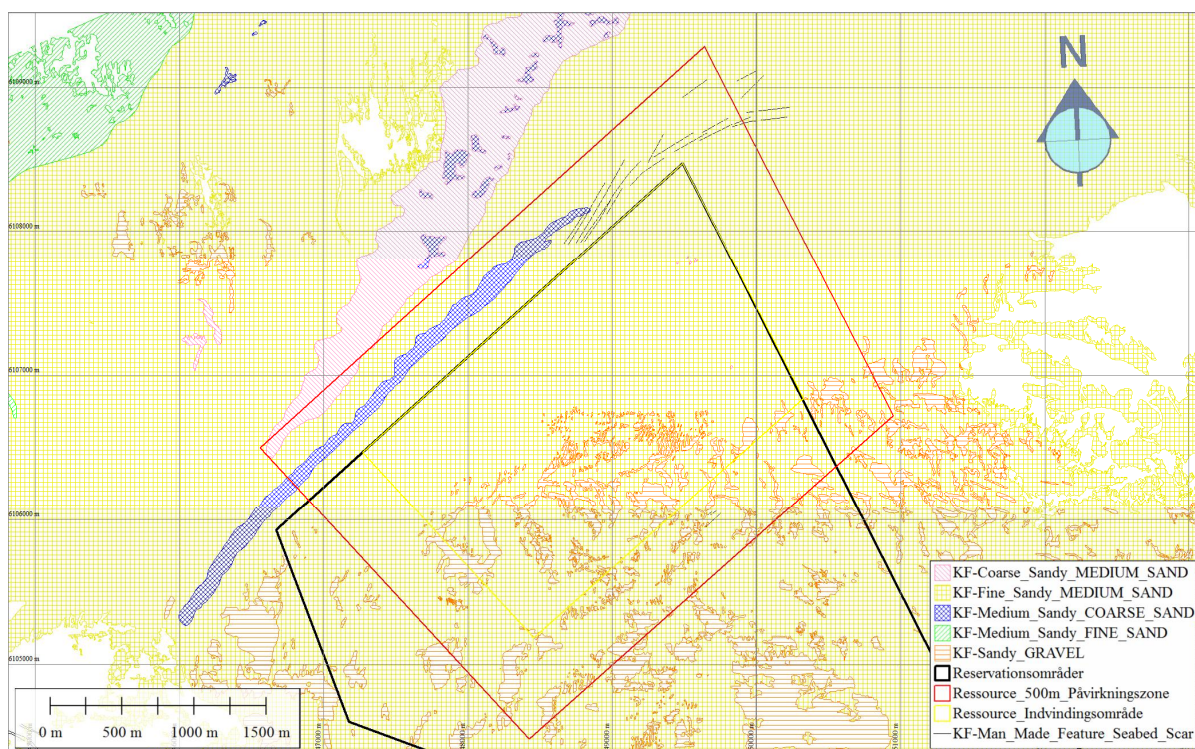
Figur 8 Oversigt over overfladesedimentkort udarbejdet under tolkning af Kriegers Flak OWF, 2013
