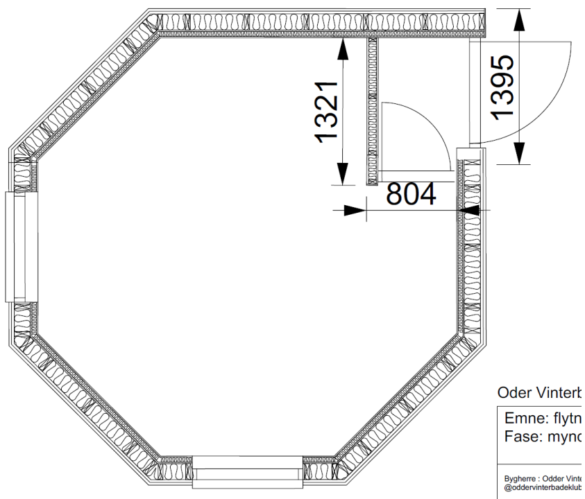
Fig. 5. På figuren ses en tegning af den ansøgte ændrede entré på saunabygningen.
