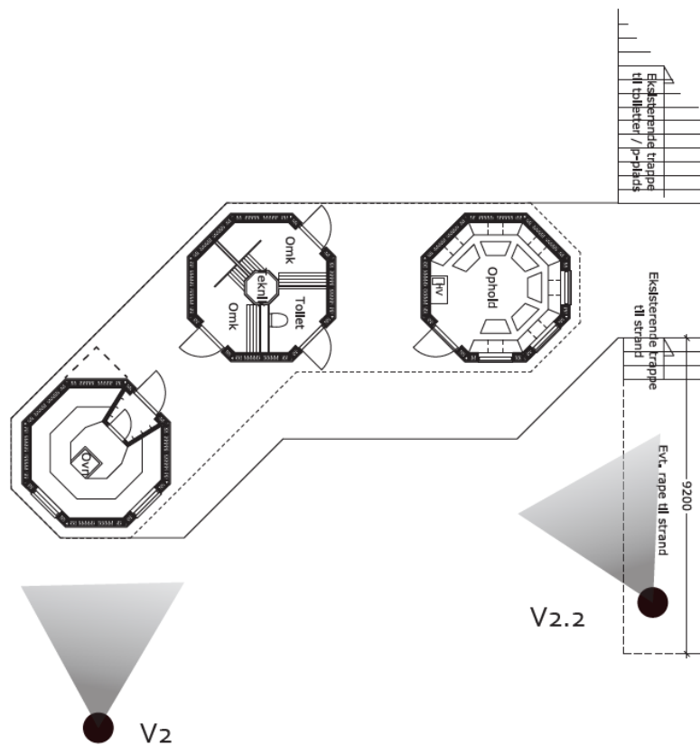
Fig. 7. Tilsendt fra ansøger. På figuren ses en plantegning over den eksisterende badeanstalt. Den ansøgte ændring af saunaens entré er markeret med en stiple sort linje. Et billede taget fra V2 og V2.2 ses på de efterfølgende figurer (8 og 9).
