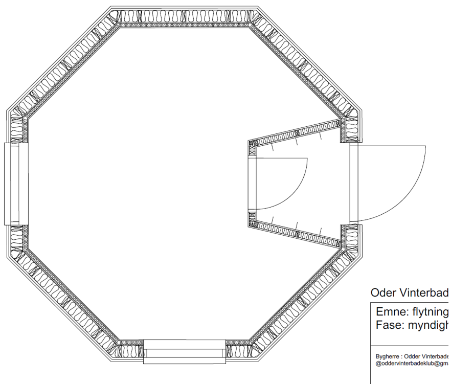
Fig. 3. Tilsendt fra ansøger. På figuren ses en tegning af den nuværende saunabygning.
