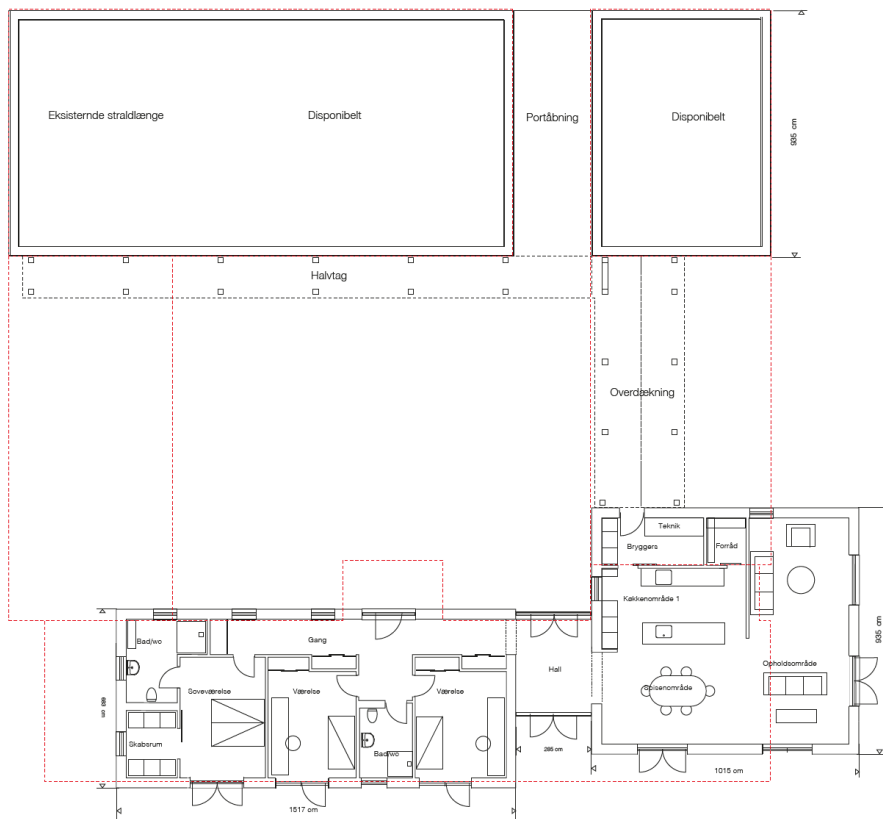
Grundplan for ansøgte forhold
