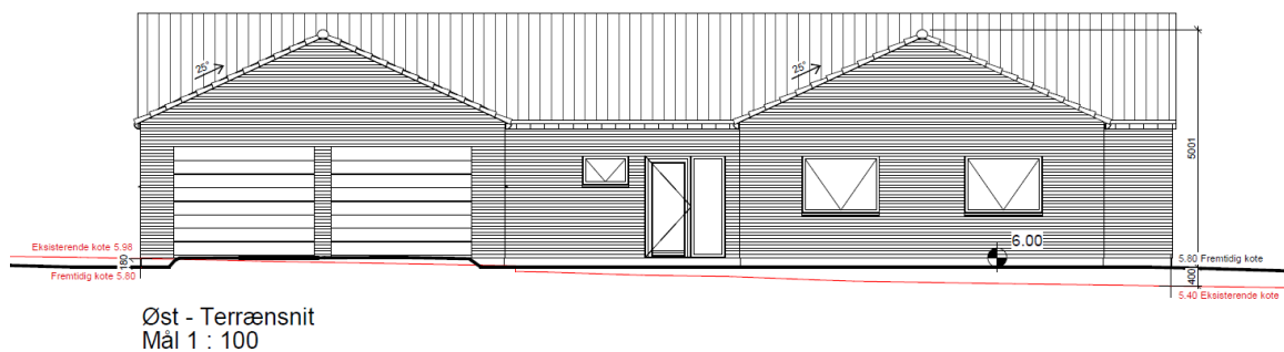
Fig. 3. facade-træsnit nord & øst. Solceller placeret på det nordvendte tag, der ikke er synlige fra øst.
