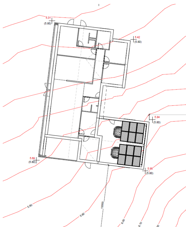
Fig. 4. Situationsplan, med opmarkering af fladerne for solcellerne. Ansøger oplyser, at der i løsningen er vægtet symmetri for et mere harmonisk udtryk.
