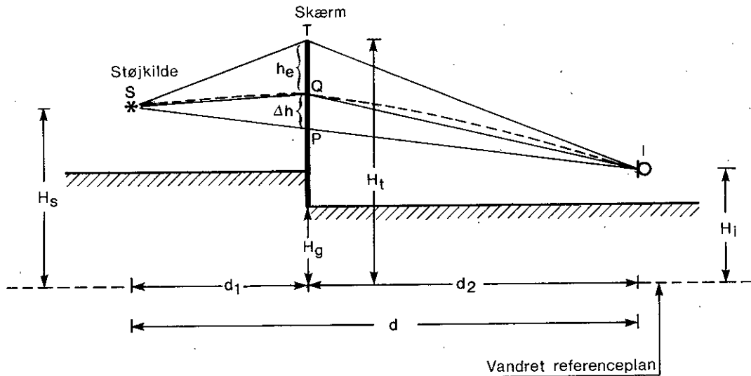
Figur 5.3.5 Lodret snit gennem kilde og beregningspunkt med nogle af de størrelser, der bruges ved beregning af skærmskorrektionen \Delta L_s .
