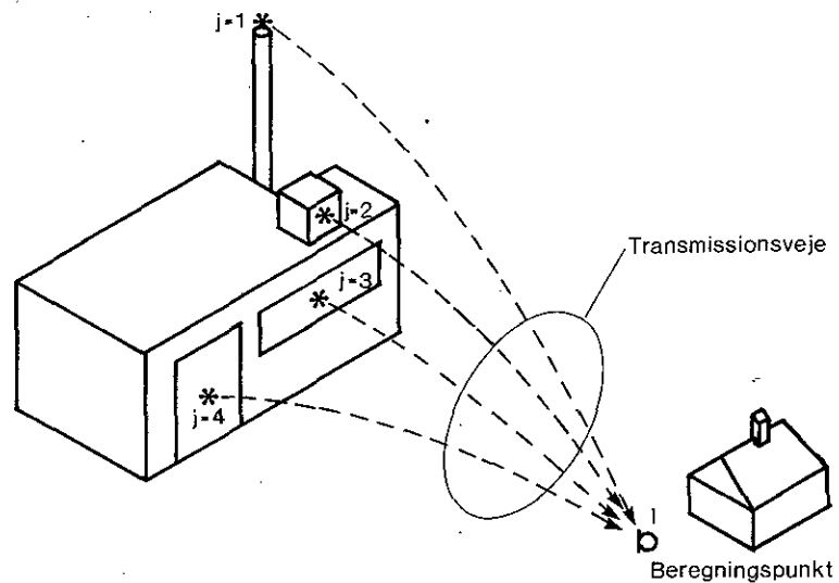
Figur 5.1.1 Beregningsmetodens struktur. I eksemplet er der fire støjkilder med numrene j=1...4 .
