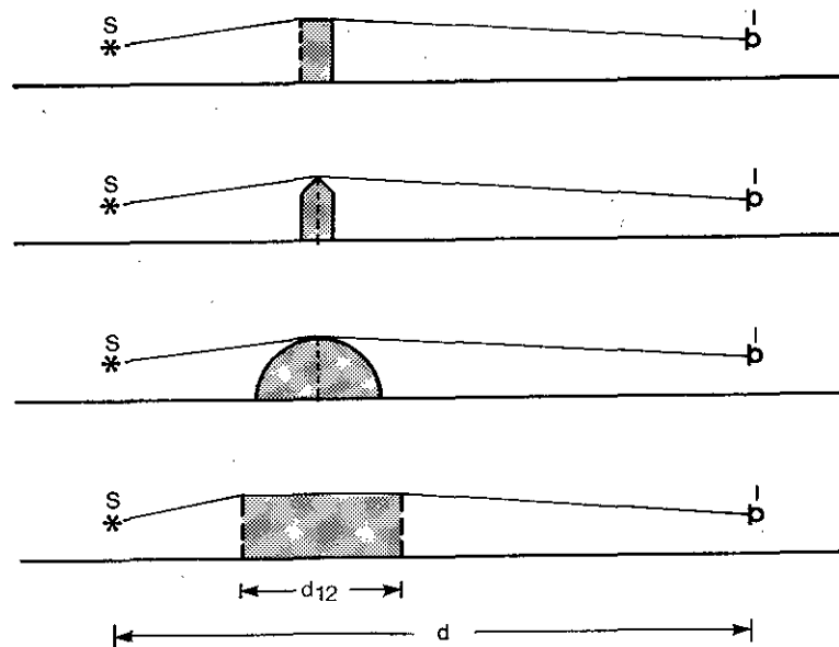
Figur 5.3.9 Eksempler på, hvordan en bygning repræsenteres ved tænkte, tynde skærme ved beregningen af \Delta L_s .
