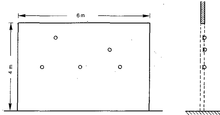
Figur 6.3.5 Opstalt og lodret snit i portåbning med angivelse af målepunkter.
