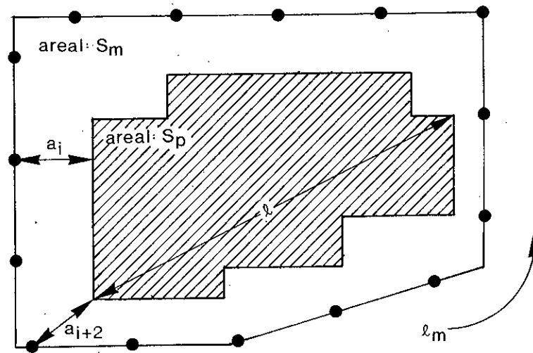
Figur 6.4.1 Illustration af begræbnerne grundflade, S_p , og målelimens fladeindhold, S_m .
