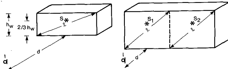
Figur 5.2.3 Opdeling af en bygningsfacade i delkilder, som hver overholder kriteriet l < d .
