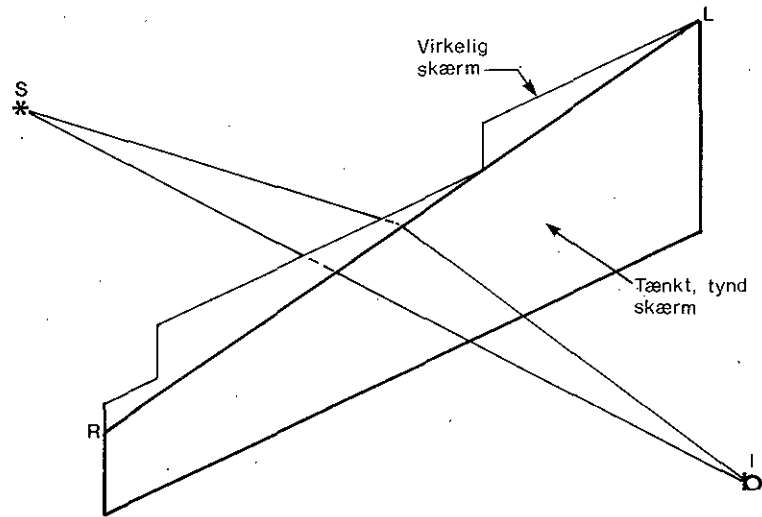
Figur 5.3.8 Tænkt, tynd skærm, der repræsenterer de virkelige skærm ved beregningen.
