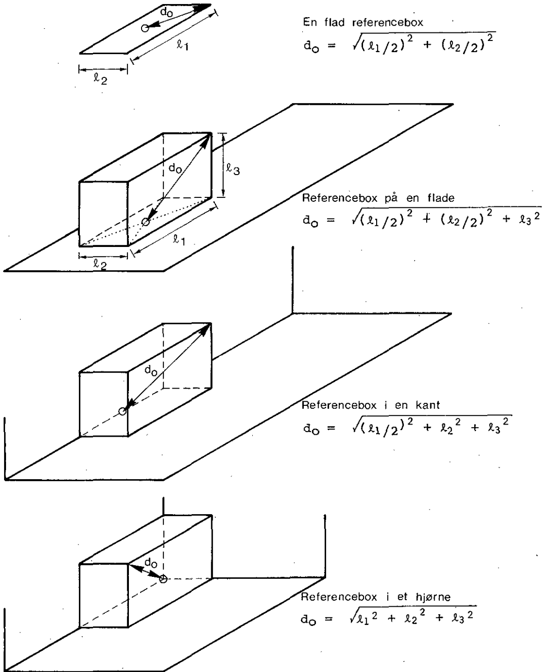
Figur 6.1.2 Eksempler på referencebokse og angivelse af karakteristisk dimension, d_o
