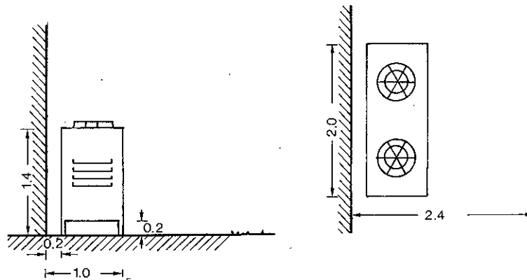
Figur 6.3.3 Opstalt og plan af køleaggregat og opstillet uden for fabriksbygning. Alle mål i meter.
