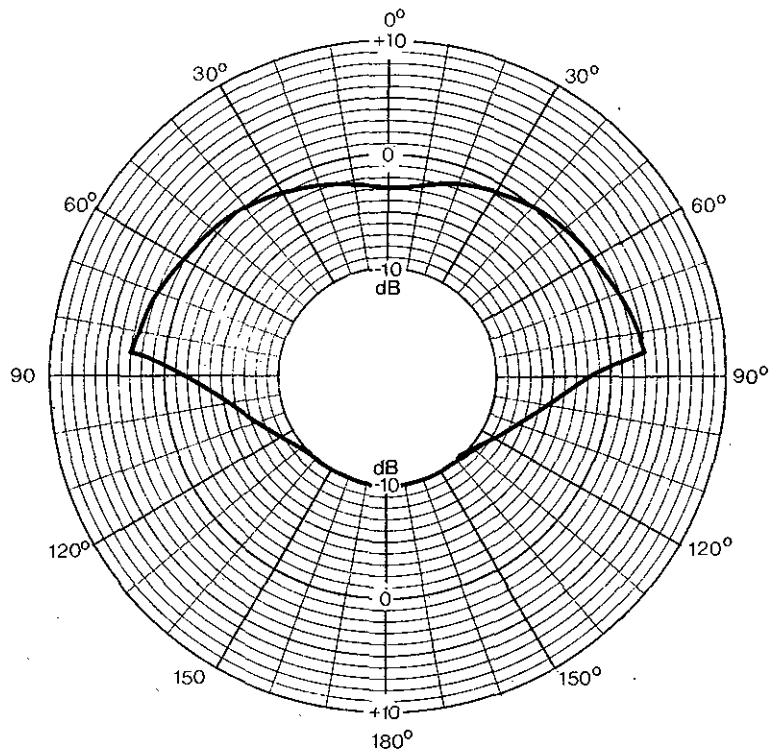
Figur 7.2.3 Retningskorrektions for bygningsdele.
