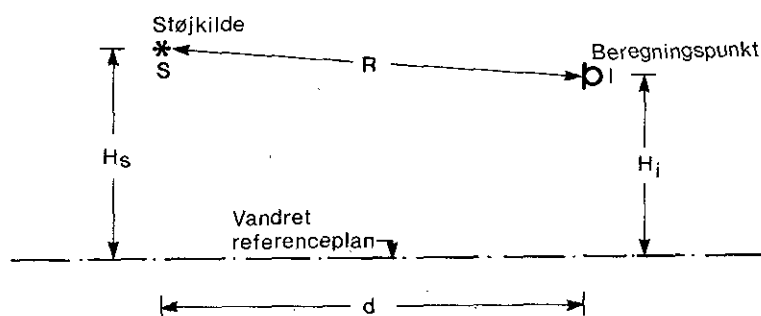
Figur 5.3.1 Lodret snit gennem kilde og beregningspunkt.
